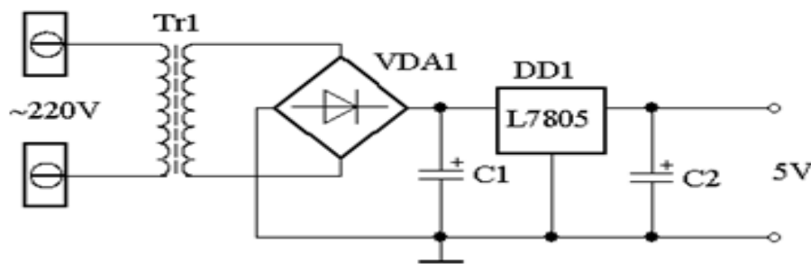
Рисунок 2.1- Схема стабілізації живлення для цифрових пристроїв на основі мікроконтролерів
