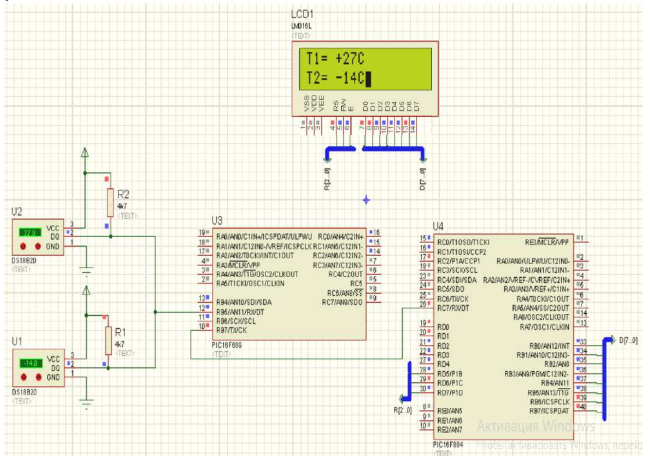
Рисунок 3.2 - Робоча схеми в PROTEUS
