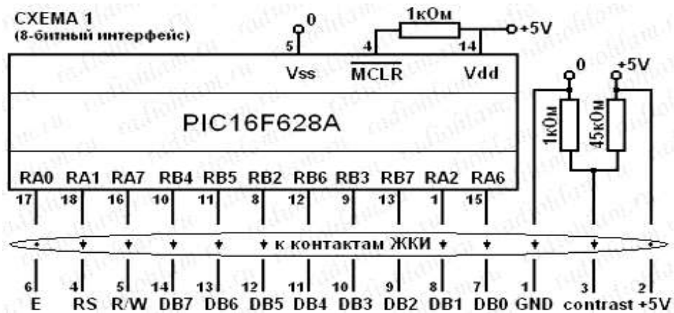
Рисунок 1.5 - Схема спряження МК з РКІ
