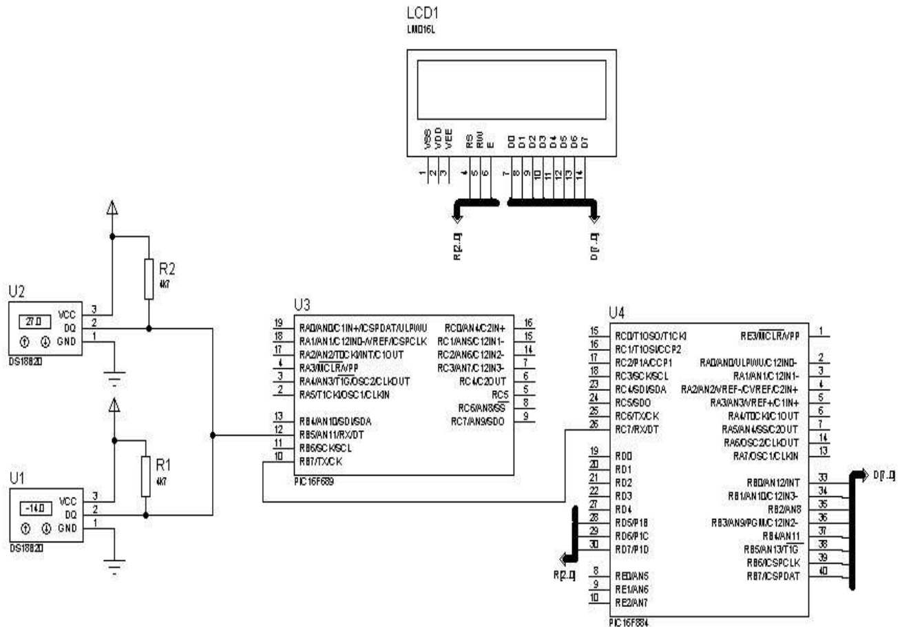
Рисунок 2.7 - Досліджувана схема
