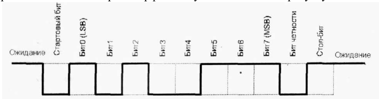
Рисунок 1.7 - Часова діаграма передачі байта E5h (11100101b).
