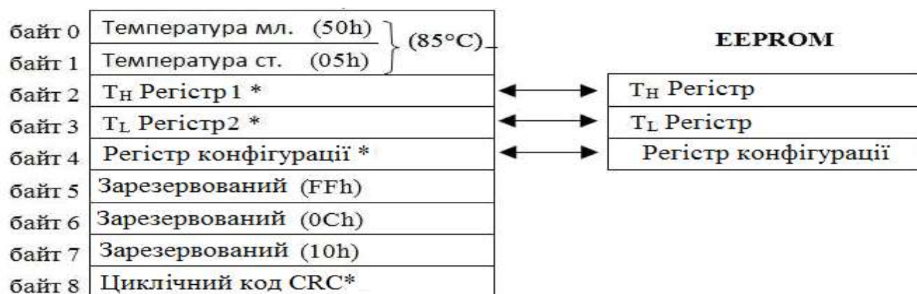
Рисунок 1.3 - Карта пам'яті DS18B20
