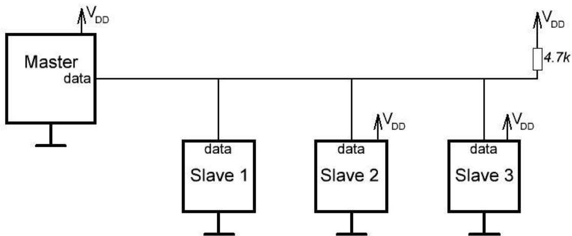
Рисунок 1.8 - Приклад підключення ведучого і ведених приладів за протоколом 1-Wire
