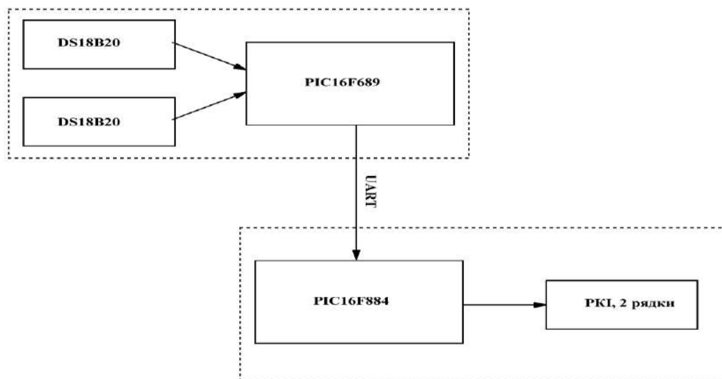
Рисунок 1.1 - Структурна схема системи моніторингу температури
