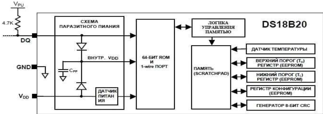
Рисунок 1. Блок-схема DS18B20
