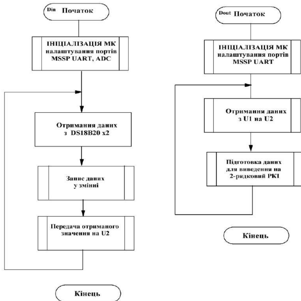
Рисунок 3.1 - Блок-схеми роботи Система моніторингу температури
