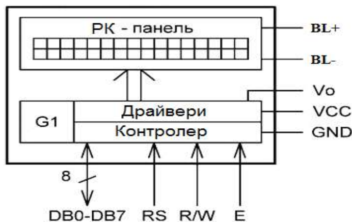
Рисунок 1.4 – Структурна схема РКІ
