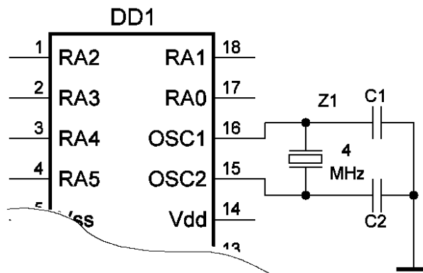
Рисунок 2.2 - Схема тактування мікроконтролера
