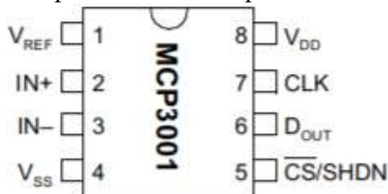
Рисунок 1.8 - Розпіновка приладу MCP3001
