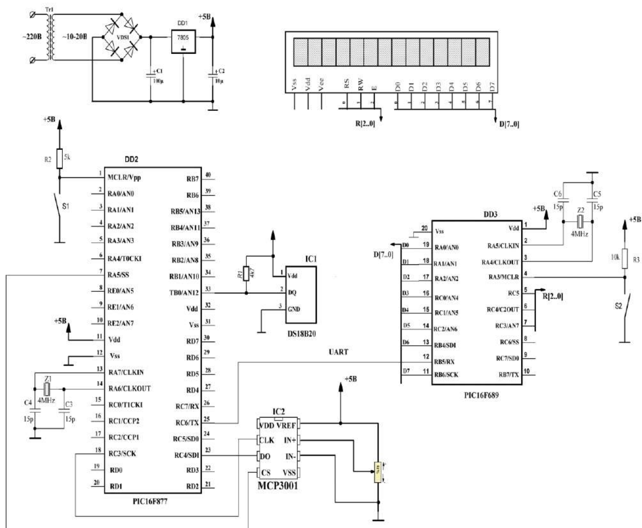
Рисунок 2.3 - Електрична принципова схема роботи Система моніторингу U та T
