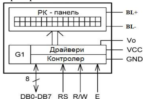
Рисунок 1.4 – Структурна схема РКІ
