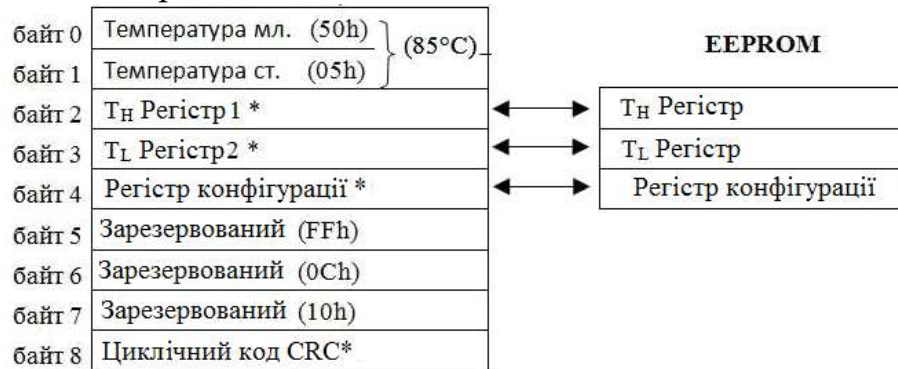
Рисунок 1.3 - Карта пам'яті DS18B20
