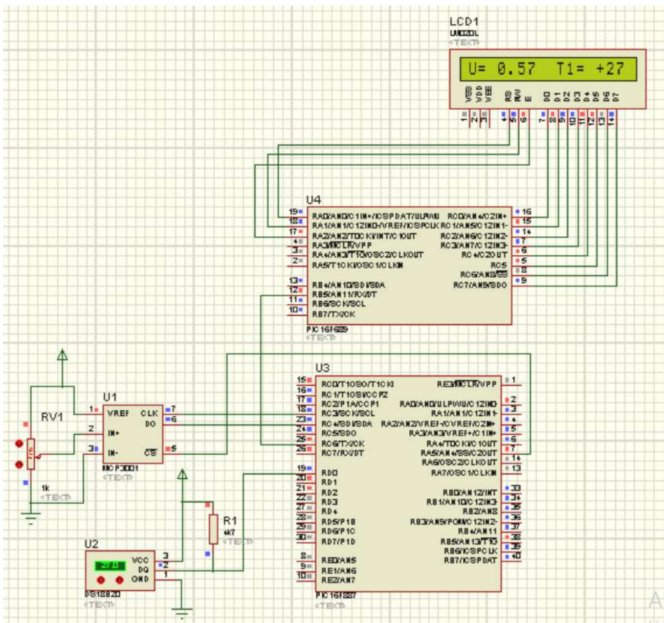
Рисунок 3.2 - Робоча схеми в PROTEUS
