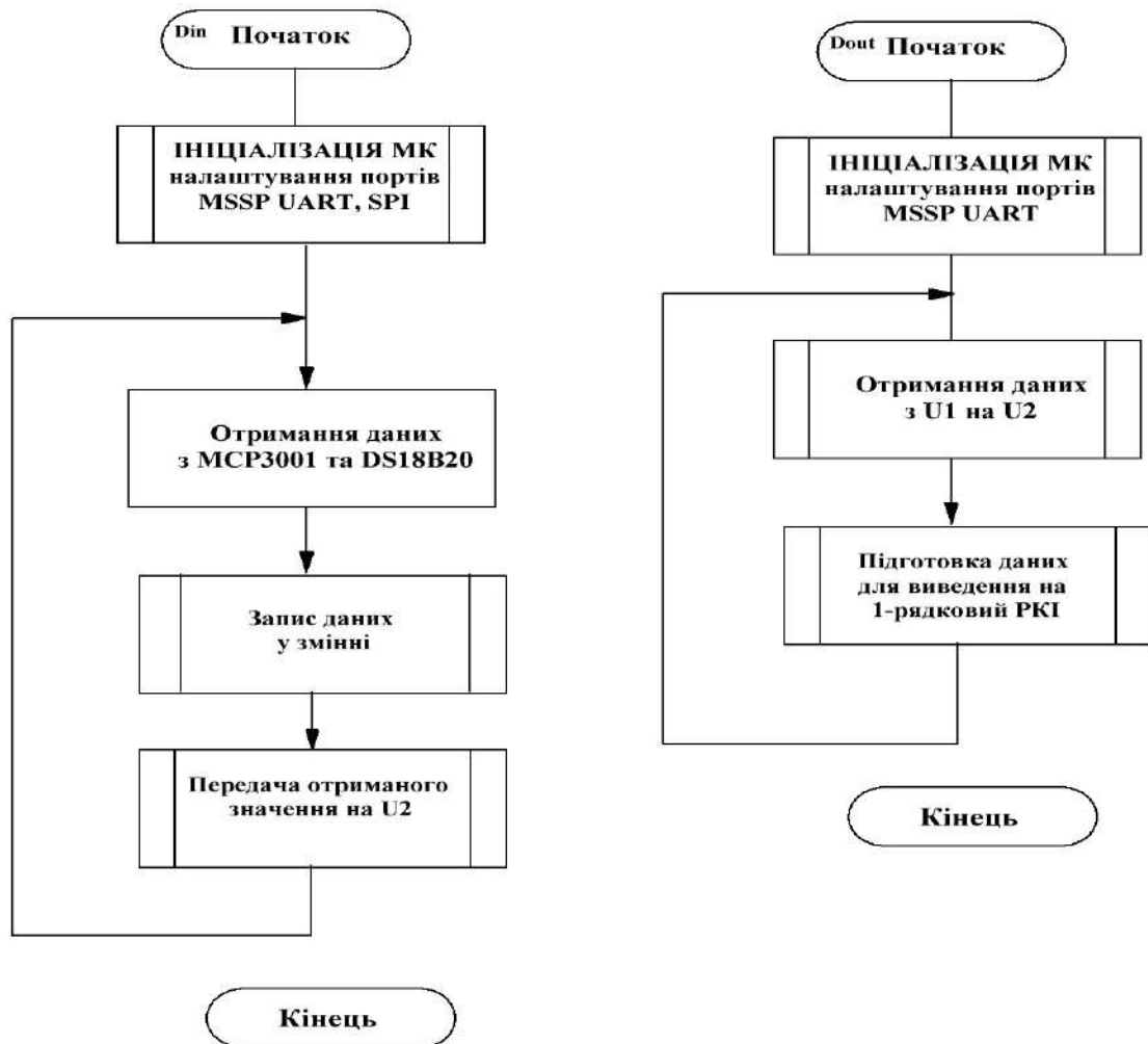
Рисунок 3.1 - Блок-схеми роботи Система моніторингу U та T
