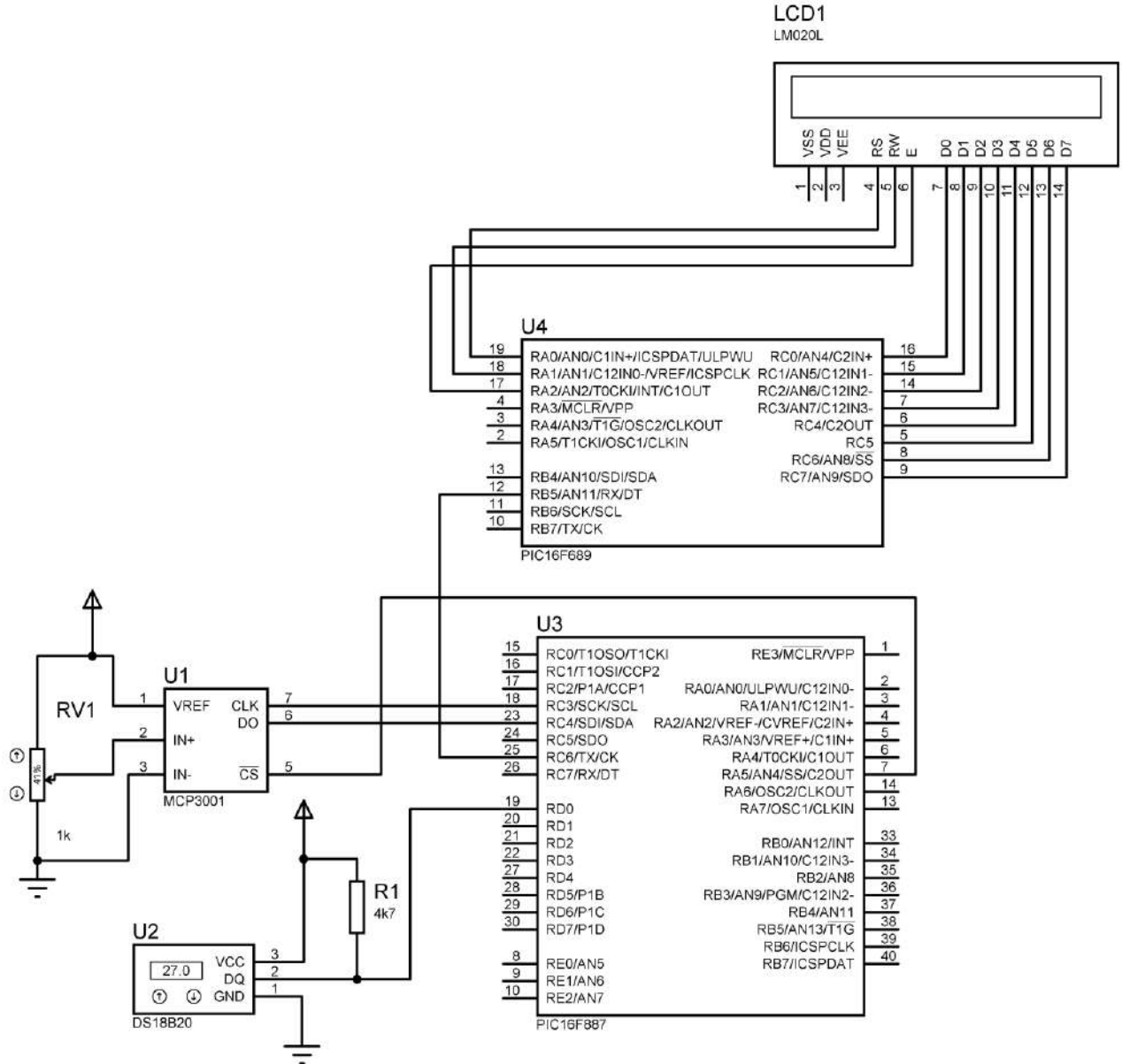
Рисунок 2.7 - Досліджувана схема
