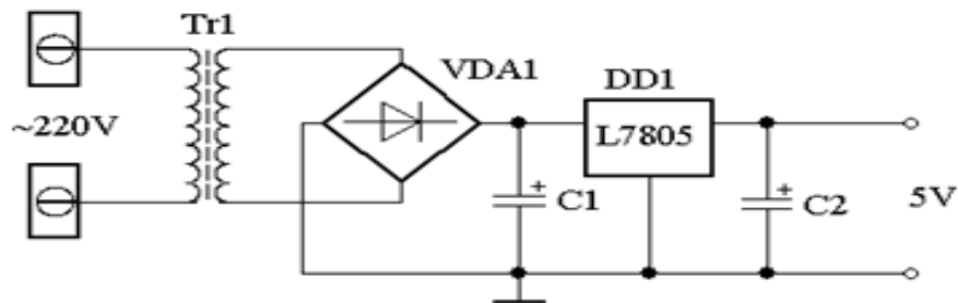
Рисунок 2.1- Схема стабілізації живлення для цифрових пристроїв на основі мікроконтролерів
