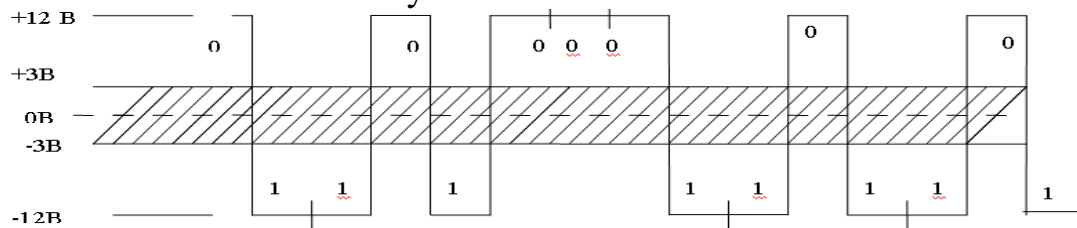
Рисунок 1.5 - Реалізація інтерфейсу RS-232 на фізичному рівні
