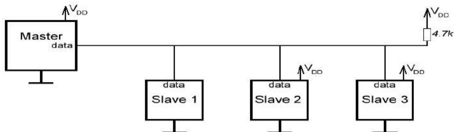
Рисунок 1.7 -Приклад підключення ведучого і ведених приладів за протоколом 1-Wire
