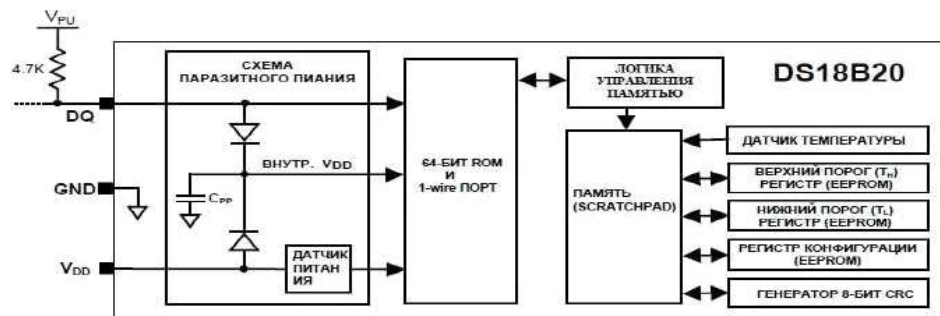
Рисунок 1.2- Блок-схема DS18B20
