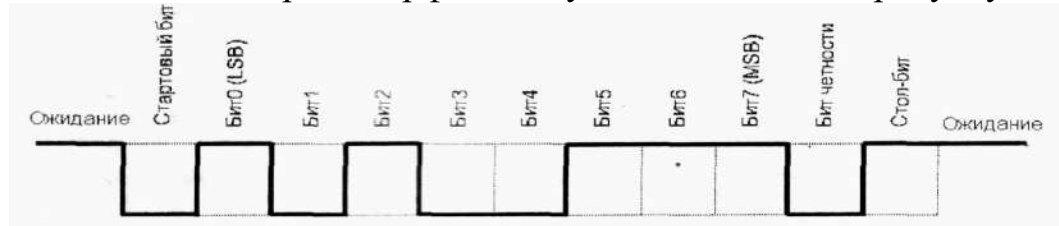
Рисунок 1.6 - Часова діаграма передачі байта E5h (11100101b).
