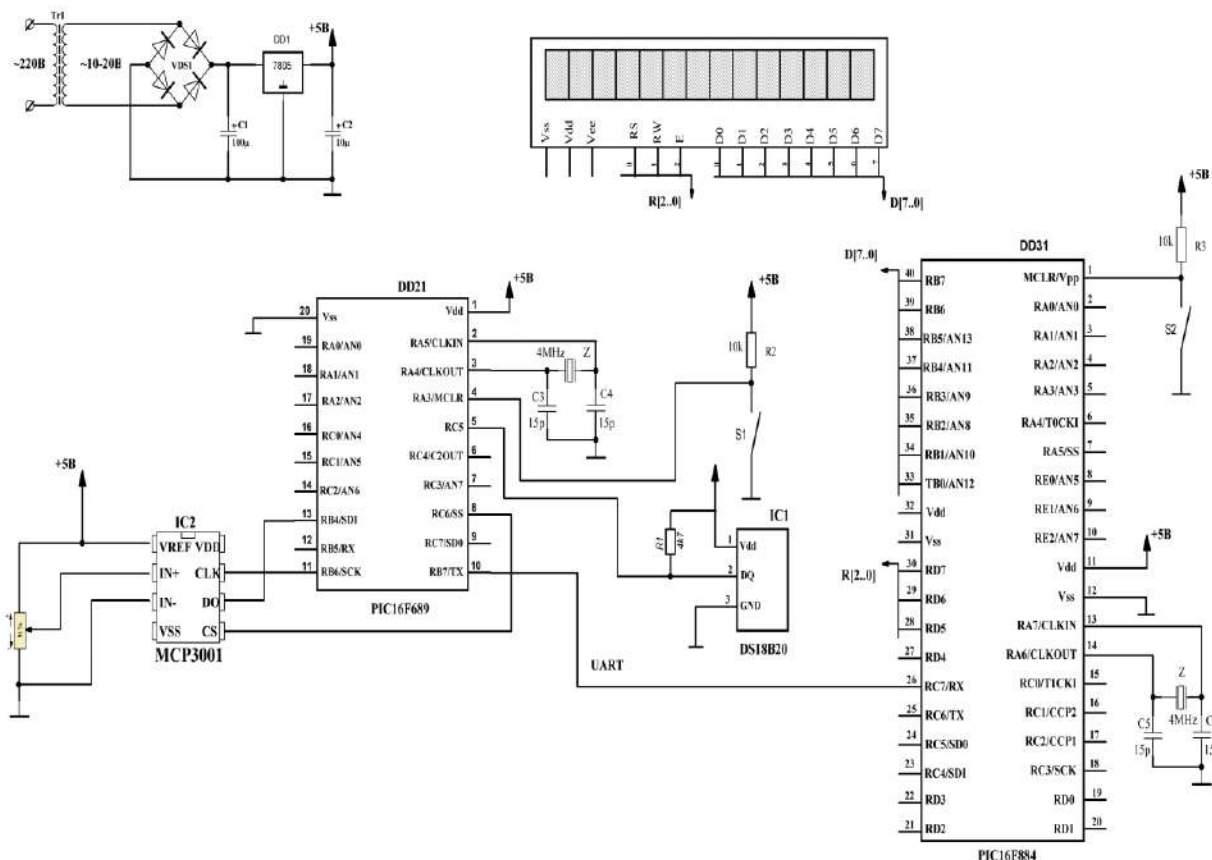
Рисунок 2.3 - Електрична принципова схема роботи Система моніторингу U та T
