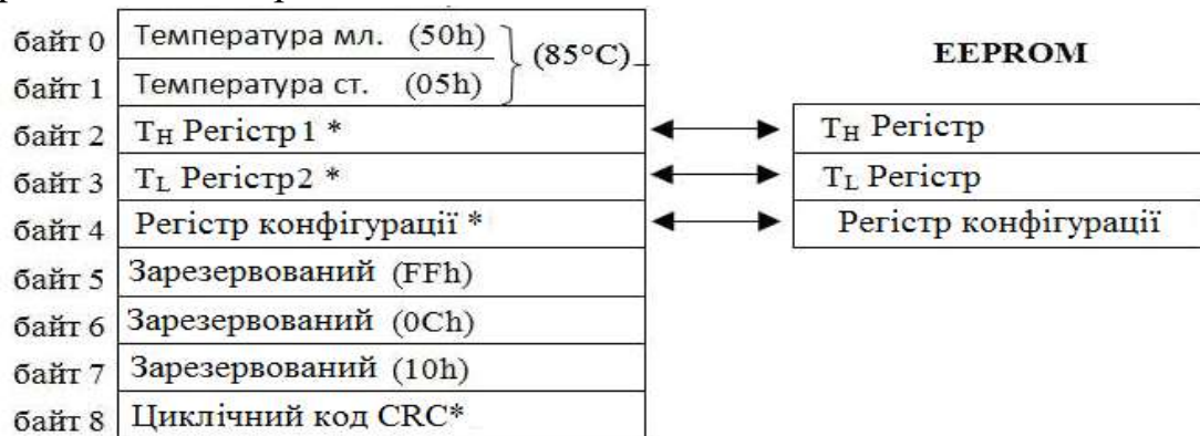
Рисунок 1.3 - Карта пам'яті DS18B20
