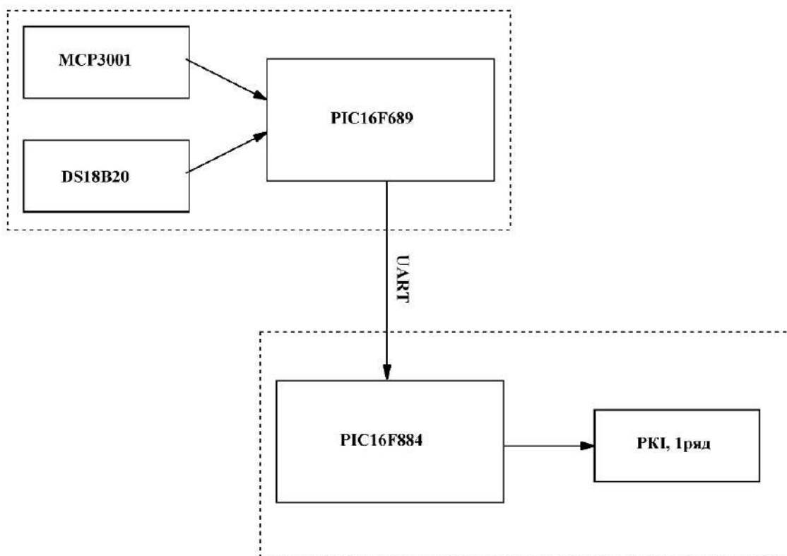
Рисунок 1.1 - Структурна схема Система моніторингу U та T
