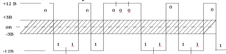
Рисунок 1.5 - Реалізація інтерфейсу RS-232 на фізичному рівні
