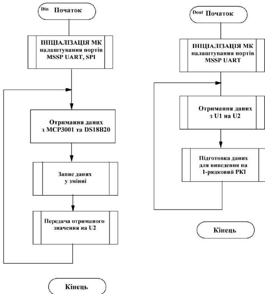
Рисунок 3.1 - Блок-схеми роботи Система моніторингу U та T
