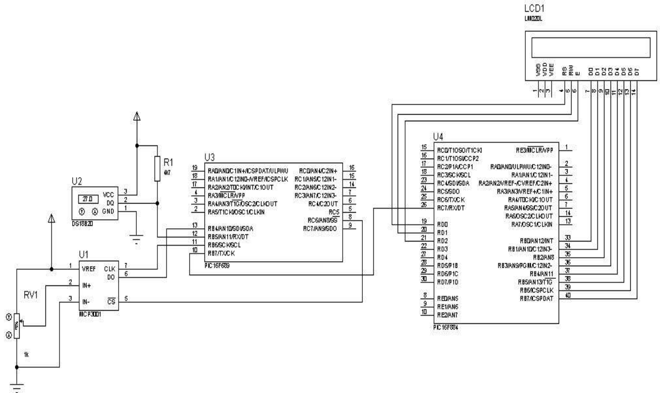
Рисунок 2.7 - Досліджувана схема
