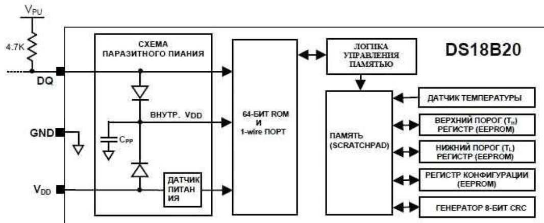
Рисунок 1.2- Блок-схема DS18B20
