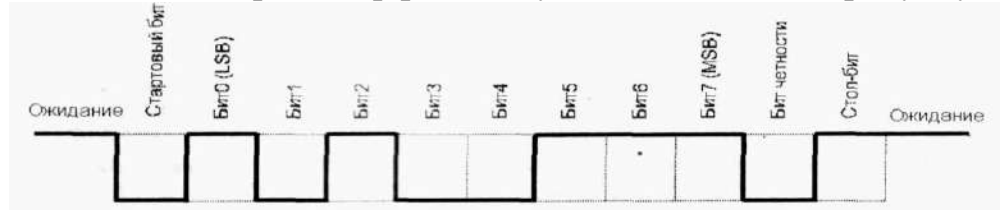
Рисунок 1.6 - Часова діаграма передачі байта E5h (11100101b).
