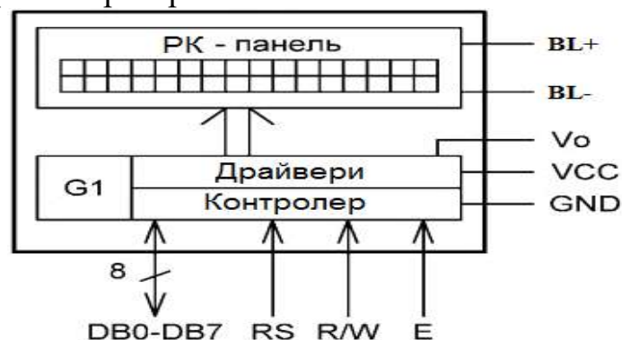
Рисунок 1.4 – Структурна схема РКІ
