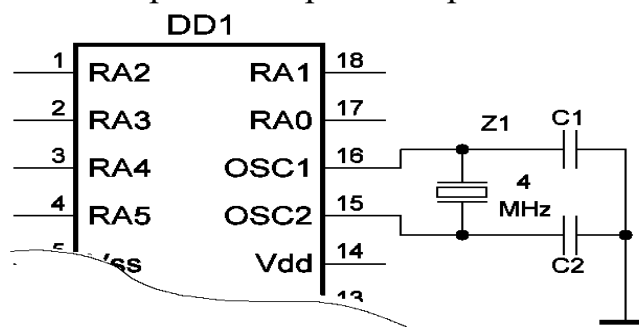
Рисунок 2.2 - Схема тактування мікроконтролера
