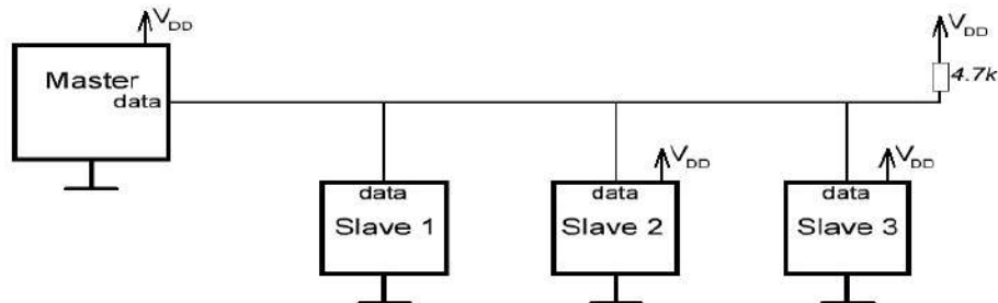
Рисунок 1.7 -Приклад підключення ведучого і ведених приладів за протоколом 1-Wire
