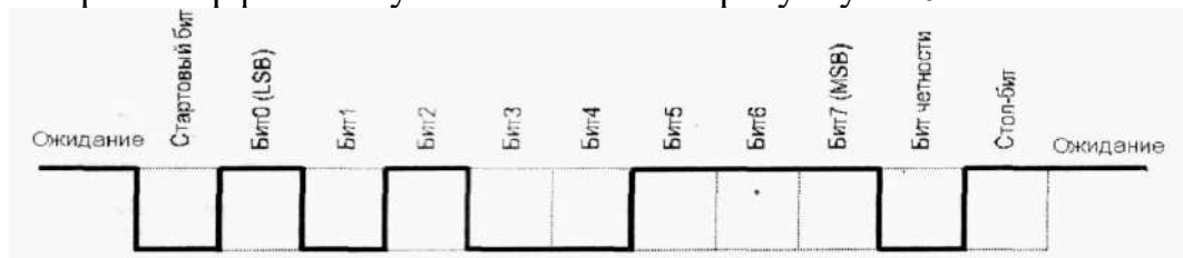
Рисунок 1.8 - Часова діаграма передачі байта E5h (11100101b).
