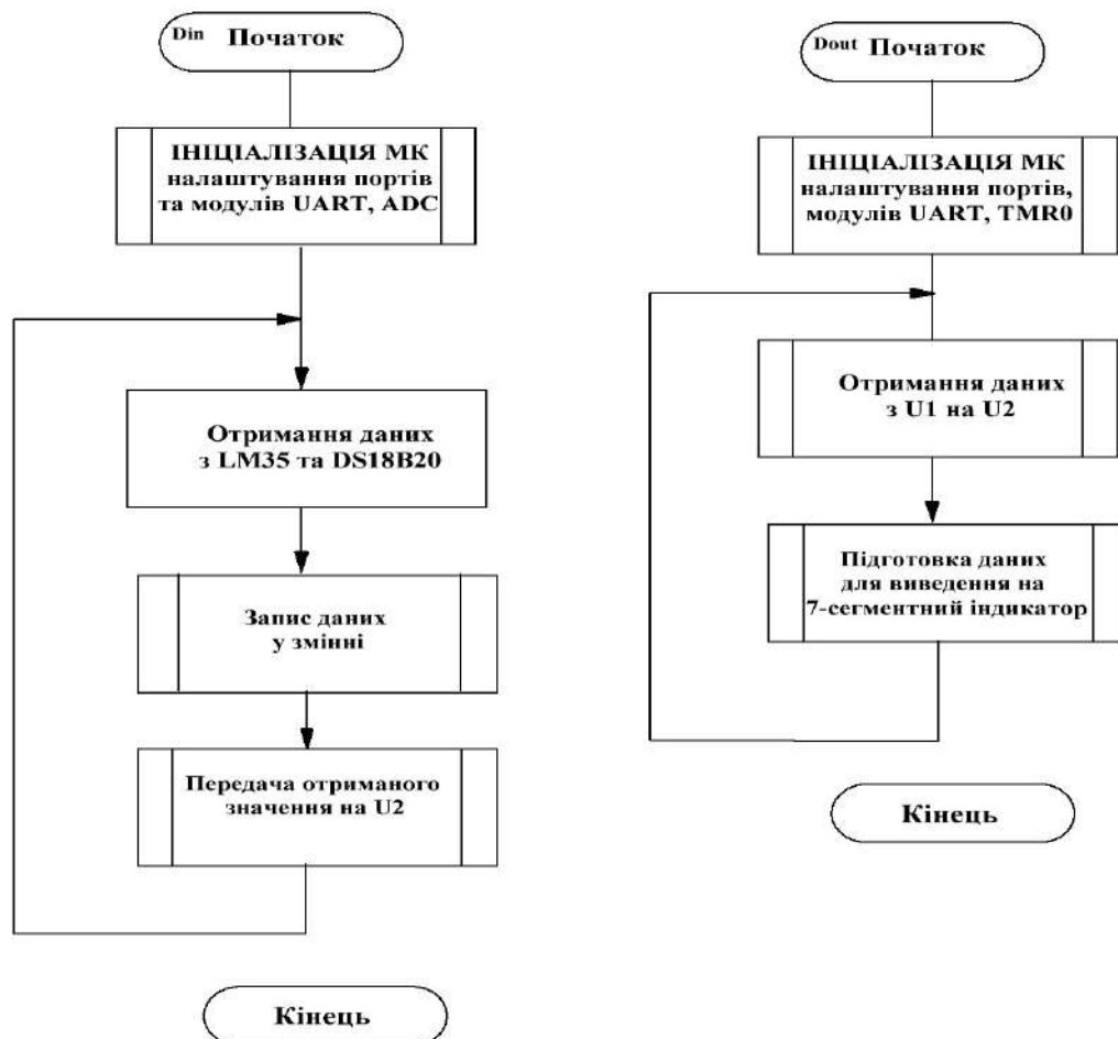
Рисунок 3.1 - Блок-схеми роботи Система моніторингу температури
