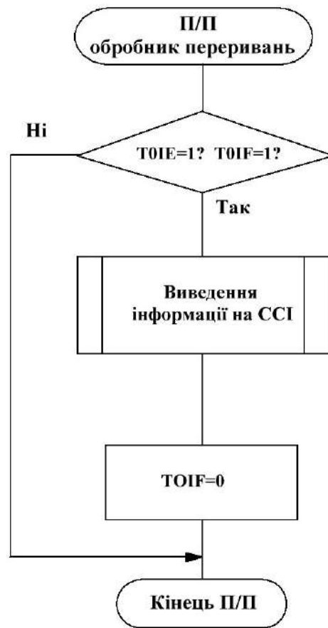
Рисунок 3.2 - Обробник переривання за TMR0
