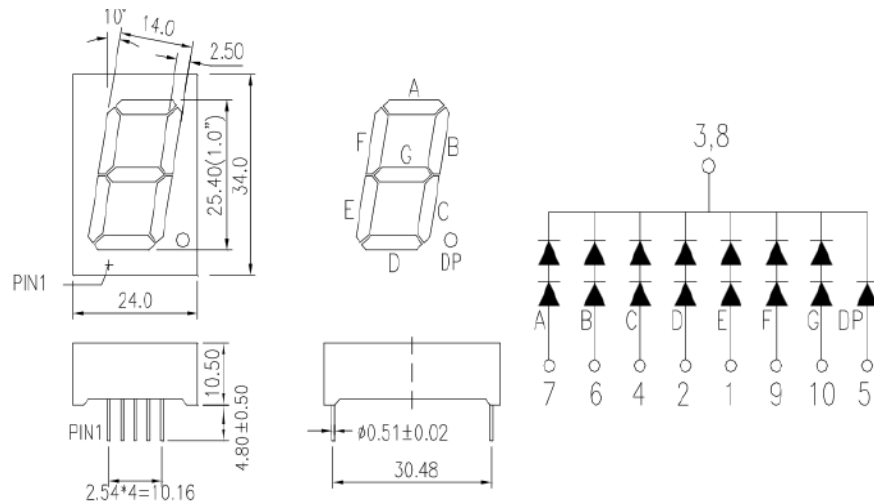
Рисунок 1.5 - Геометричні розміри та електрична схема однорозрядного ССІ зі спільним анодом.
