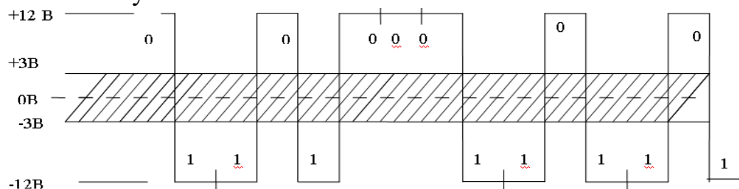
Рисунок 1.7 - Реалізація інтерфейсу RS-232 на фізичному рівні
