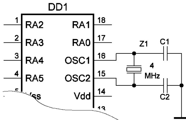
Рисунок 2.2 - Схема тактування мікроконтролера
