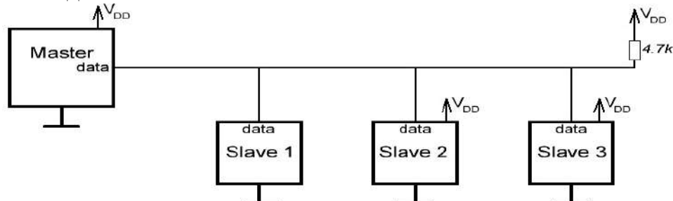
Рисунок 1.9 -Приклад підключення ведучого і ведених приладів за протоколом 1-Wire
