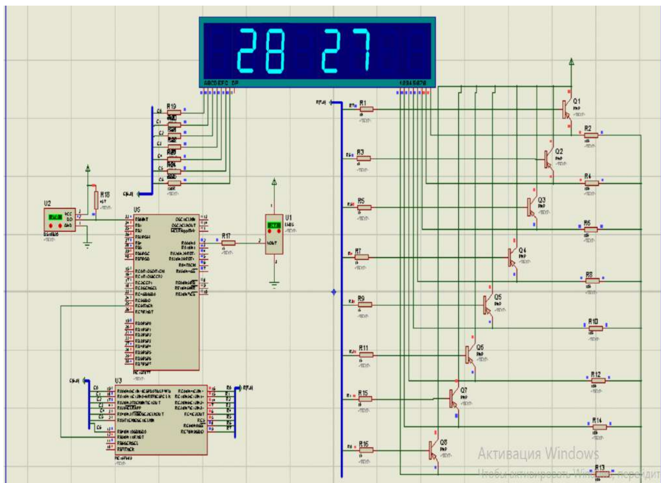
Рисунок 3.2 - Робоча схеми в PROTEUS
