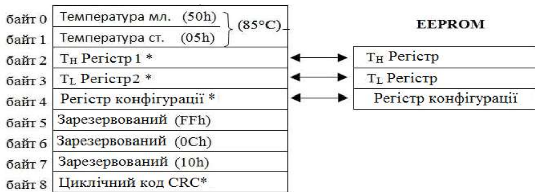
Рисунок 1.3 - Карта пам'яті DS18B20
