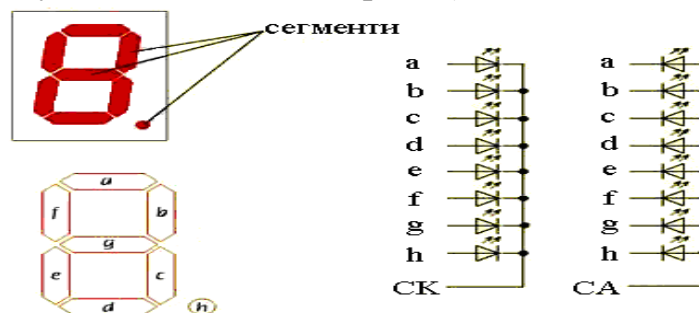
Рисунок 1.4 – Умовне графічне зображення СІІ
