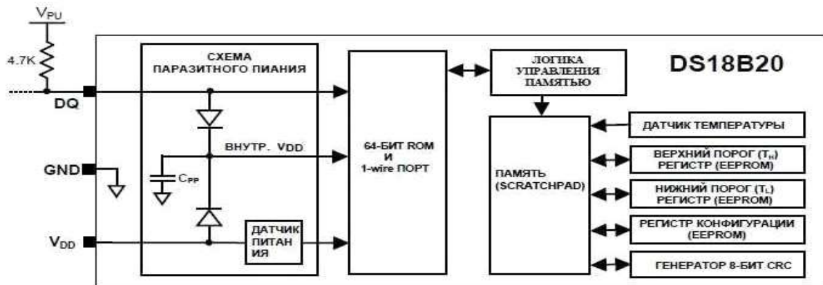
Рисунок 1.2- Блок-схема DS18B20
