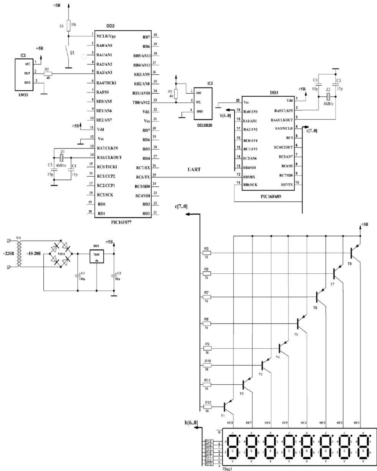
Рисунок 2.3 - Електрична принципова схема роботи Системи моніторингу температури
