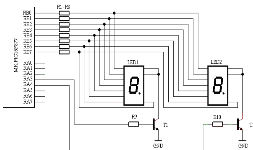
Рисунок 1.6 – Умовна схема під'єднання ССІ при динамічній індикації
