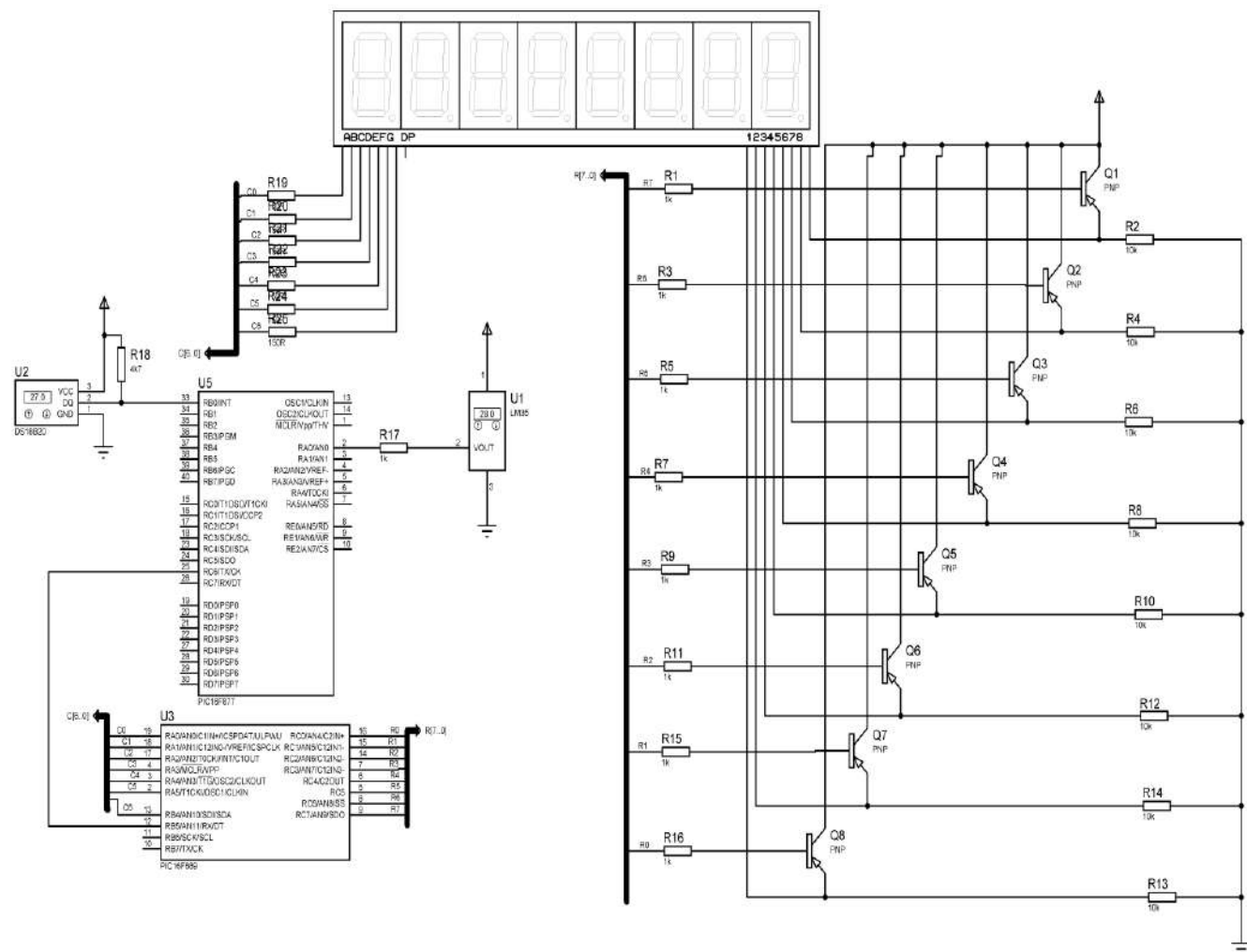
Рисунок 2.7 - Досліджувана схема
