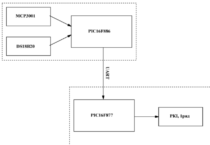
Рисунок 1.1 - Структурна схема системи моніторингу температури
