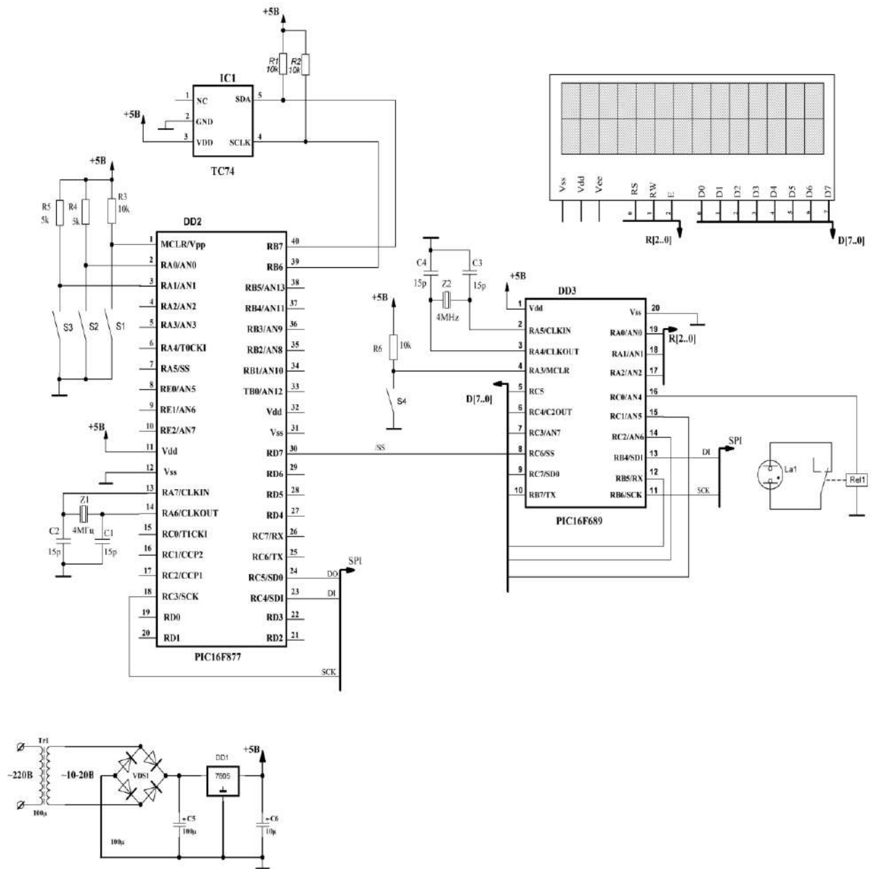
Рисунок 2.3 - Електрична принципова схема роботи Системи контролю температури
