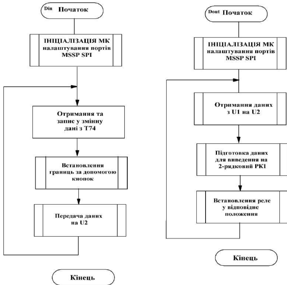
Рисунок 3.1 - Блок-схеми роботи Системи контролю температури
