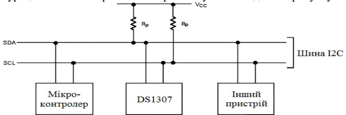
Рисунок 1.4 - Типова конфігурація двопровідної шини (I2C)
