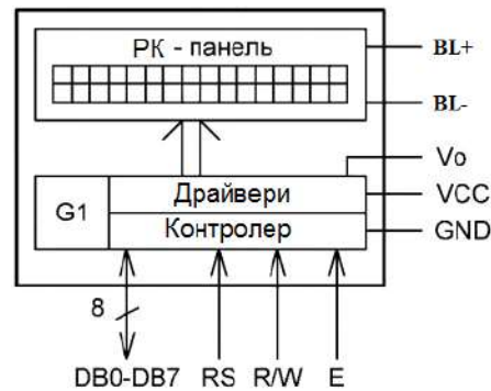
Рисунок 1.3 – Структурна схема РКІ
