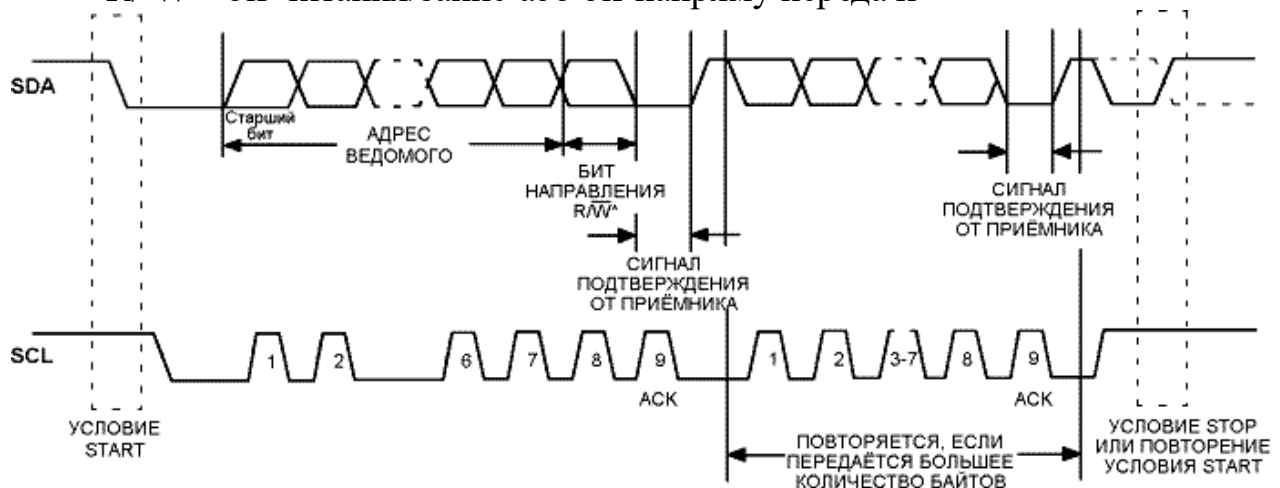
Рисунок 1.5 - Передача даних по двонаправленій шині (I2C)
