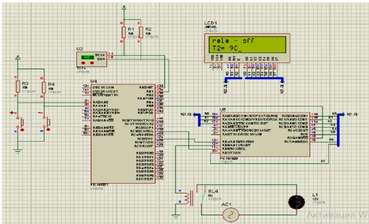
Рисунок 3.2 - Робоча схеми в PROTEUS в режимі виключеного реле
