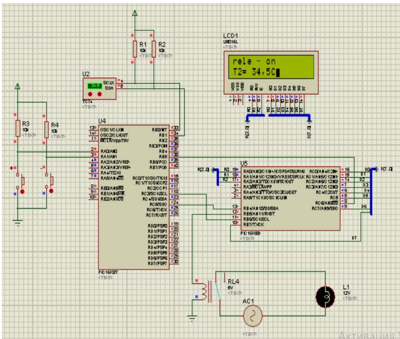
Рисунок 3.3 - Робоча схеми в PROTEUS в режимі включеного реле
