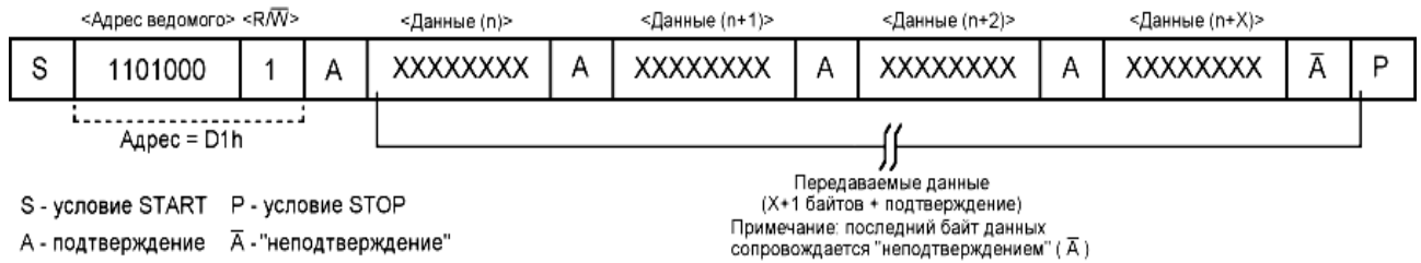
Рисунок 1.7 -Режим ведущего передатчика (режим чтения DS1307)
