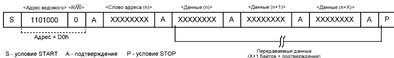
Рисунок 1.6- Режим веденого приймача(режим запису DS1307).
