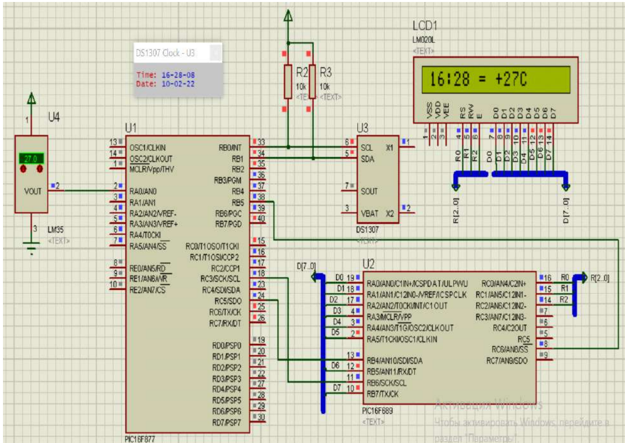
Рисунок 3.2 - Робоча схеми в PROTEUS
