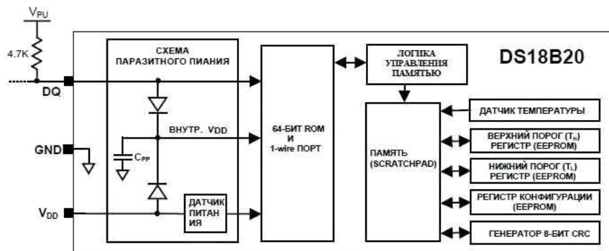
Рисунок 1.2- Блок-схема DS18B20
