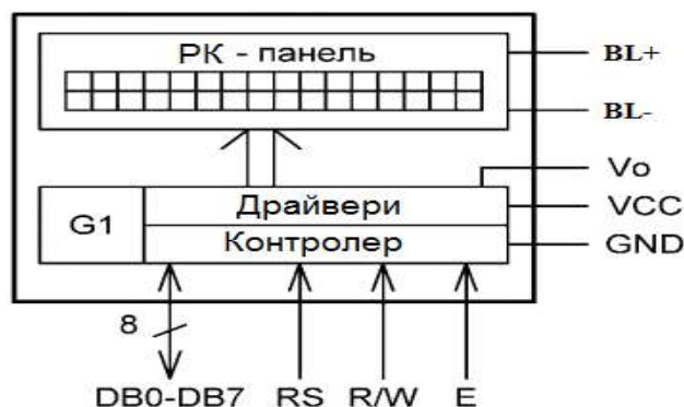
Рисунок 1.4 – Структурна схема РКІ
