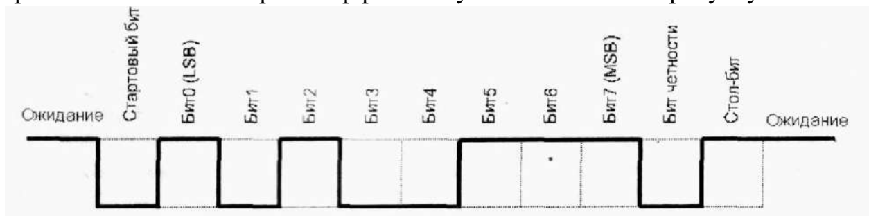
Рисунок 1.8 - Часова діаграма передачі байта E5h (11100101b).
