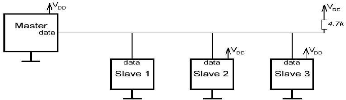
Рисунок 1.9 -Приклад підключення ведучого і ведених приладів за протоколом 1-Wire
