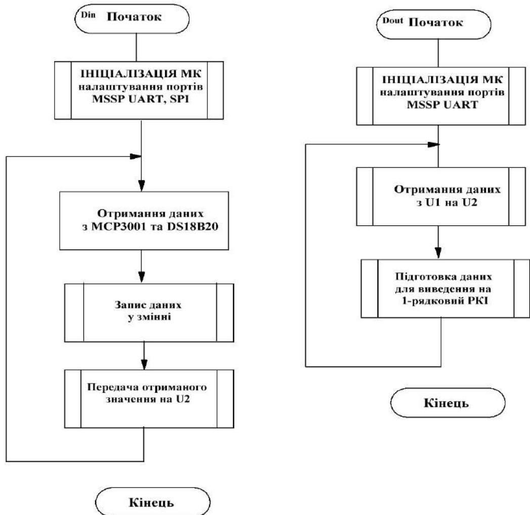
Рисунок 3.1 - Блок-схеми роботи Система моніторингу U та T
