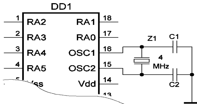
Рисунок 2.2 - Схема тактування мікроконтролера
