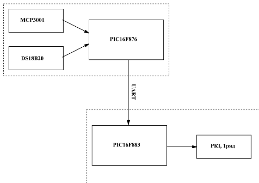
Рисунок 1.1 - Структурна схема Система моніторингу U та T
