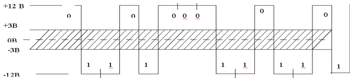
Рисунок 1.7 - Реалізація інтерфейсу RS-232 на фізичному рівні
