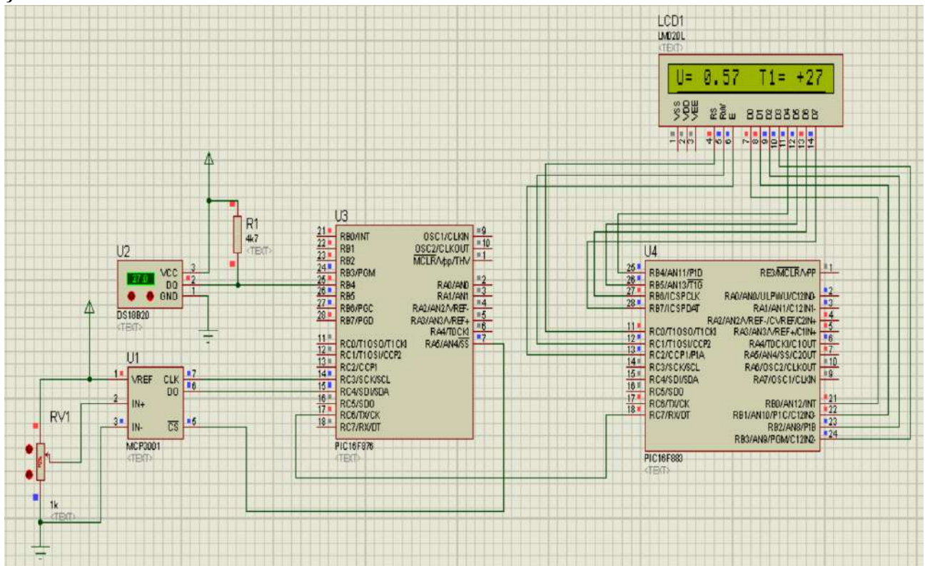
Рисунок 3.2 - Робоча схеми в PROTEUS
