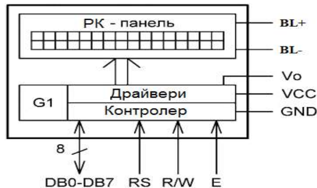
Рисунок 1.4 – Структурна схема РКІ
