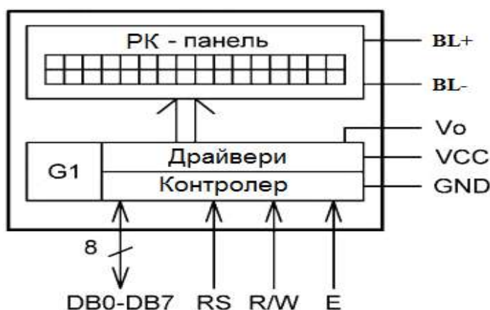
Рисунок 1.4 – Структурна схема РКІ
