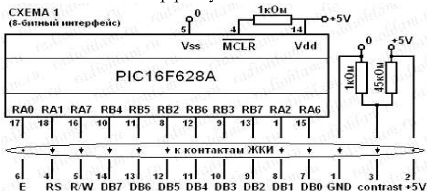
Рисунок 1.4 - Схема спраження МК з РКІ
