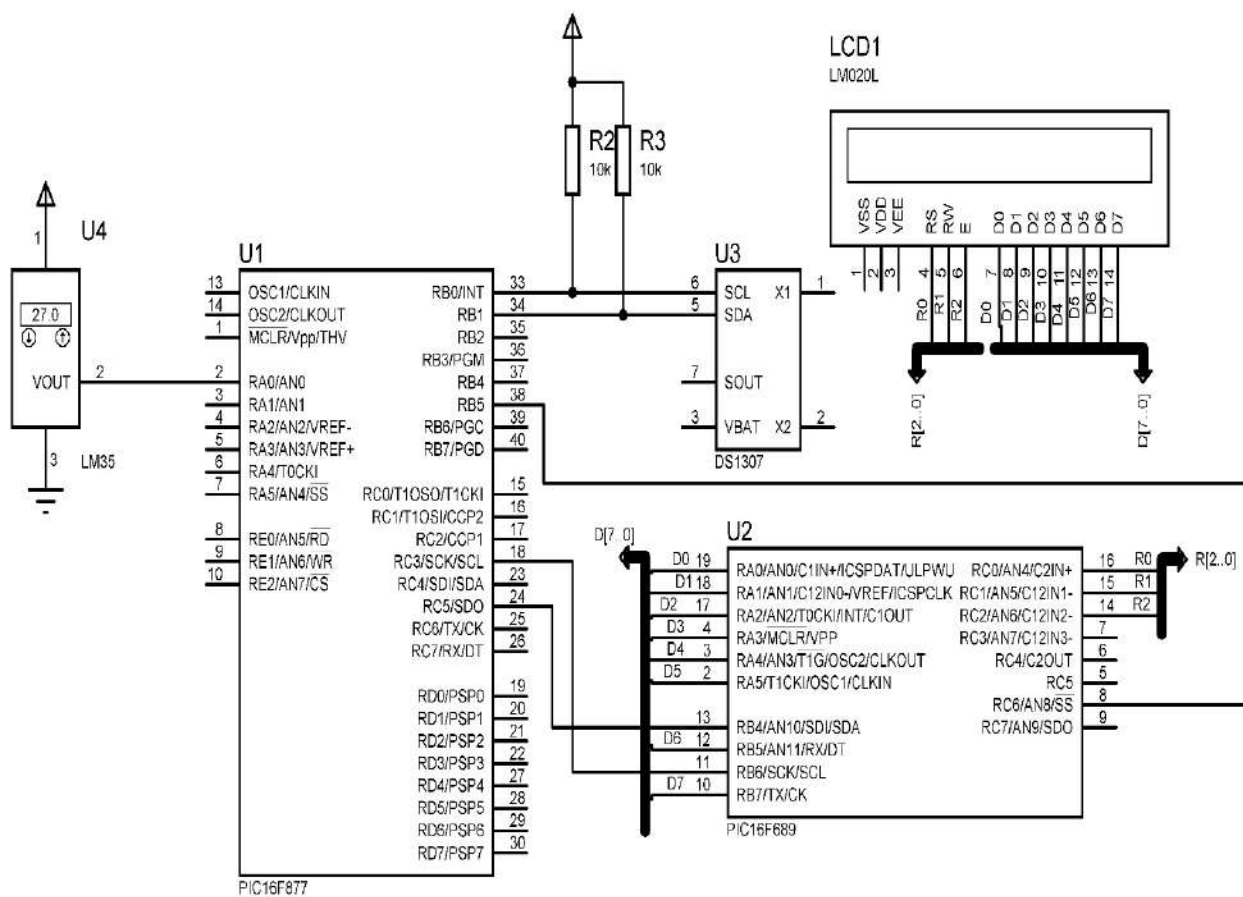
Рисунок 2.7 - Досліджувана схема
