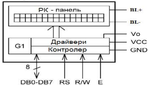
Рисунок 1.3 – Структурна схема РКІ
