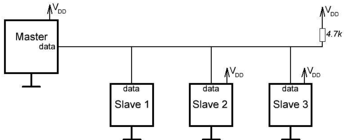
Рисунок 1.9 -Приклад підключення ведучого і ведених приладів за протоколом 1-Wire
