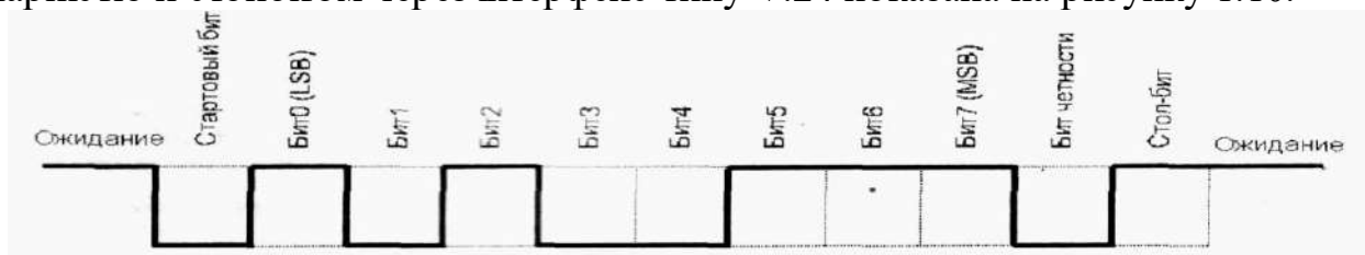
Рисунок 1.8 - Часова діаграма передачі байта E5h (11100101b).
