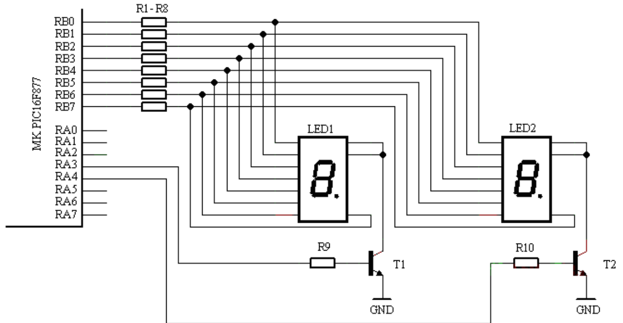
Рисунок 1.6 – Умовна схема під'єднання ССІ при динамічній індикації
