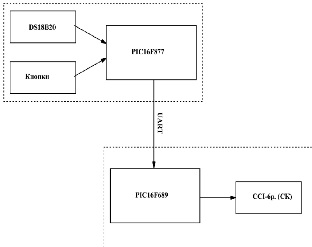
Рисунок 1.1 - Структурна схема системи контролю температури
