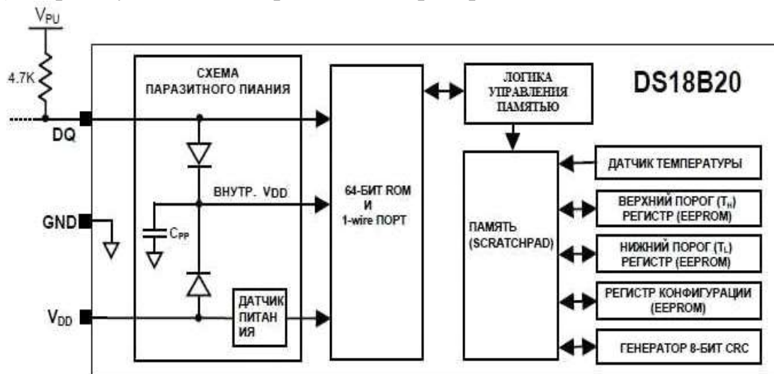
Рисунок 1.2- Блок-схема DS18B20
