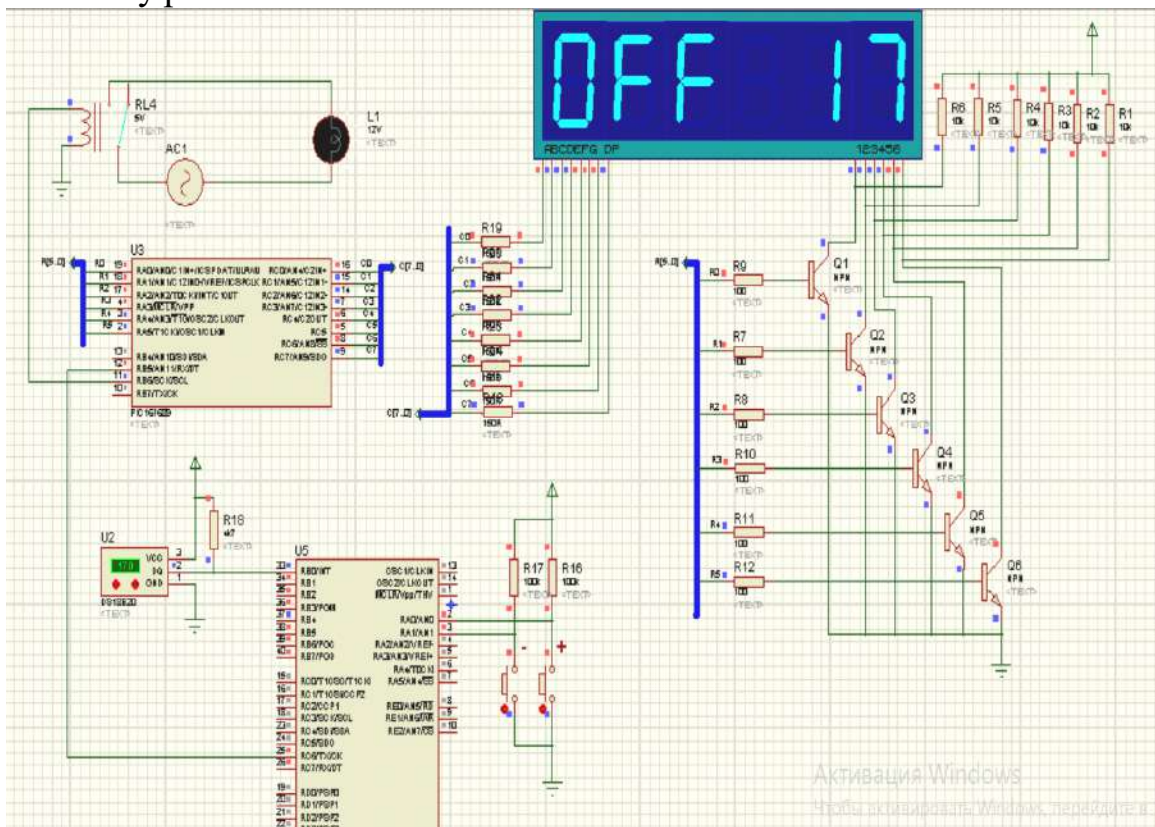
Рисунок 3.3 - Робоча схема з вимкненим реле
