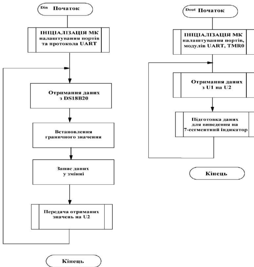
Рисунок 3.1 - Блок-схеми роботи Система контролю температури
