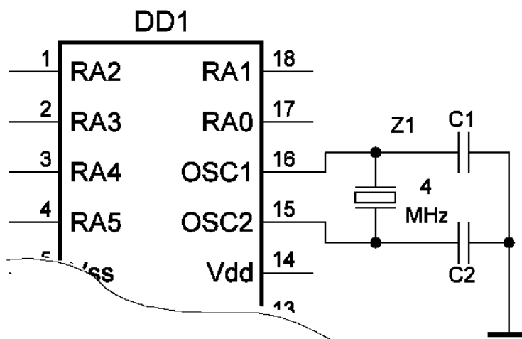
Рисунок 2.2 - Схема тактування мікроконтролера
