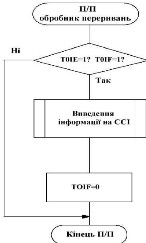
Рисунок 3.2 - Обробник переривання за TMR0
