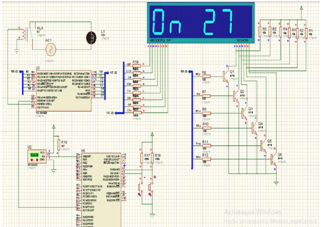
Рисунок 3.4 - Робоча схема з включенням реле
