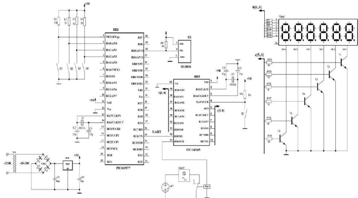
Рисунок 2.3 - Електрична принципова схема роботи Системи контролю температури
