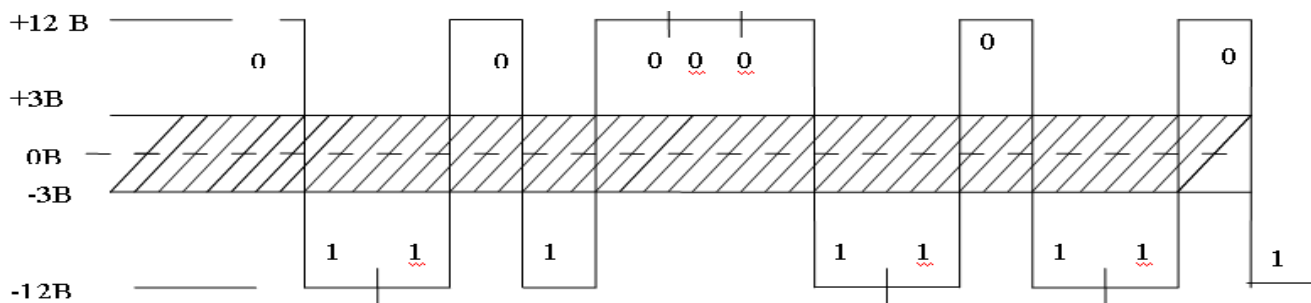
Рисунок 1.7 - Реалізація інтерфейсу RS-232 на фізичному рівні
