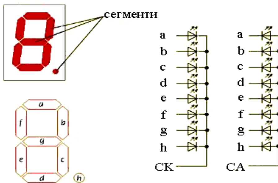
Рисунок 1.4 – Умовне графічне зображення ССІ
