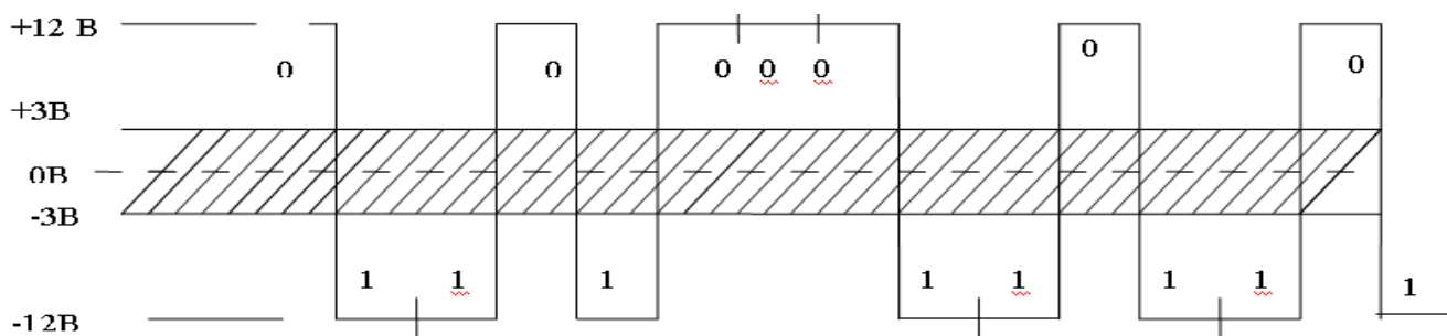
Рисунок 1.7 - Реалізація інтерфейсу RS-232 на фізичному рівні
