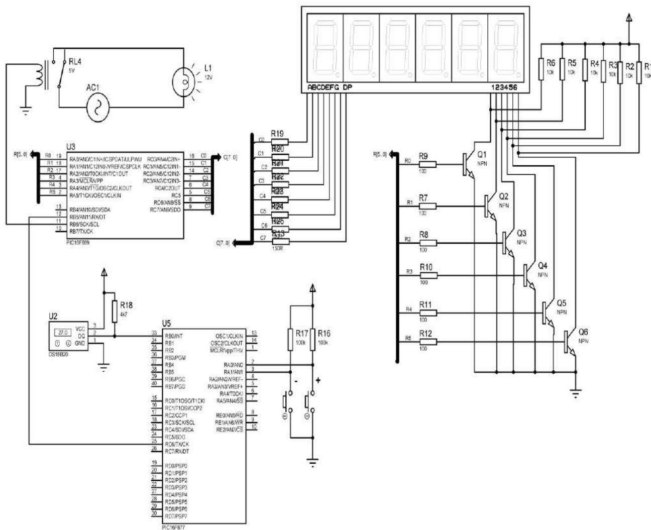
Рисунок 2.7 - Досліджувана схема
