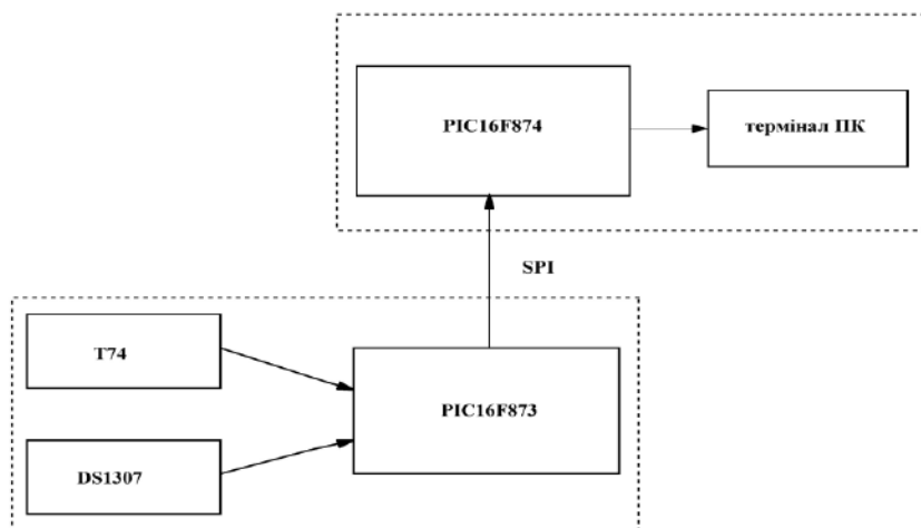
Рисунок 1.1 - Структурна схема Системи моніторингу температури
