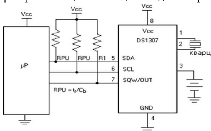
Рисунок 1.3 - Типова схема підключення модуля DS1307 до мікроконтролера
