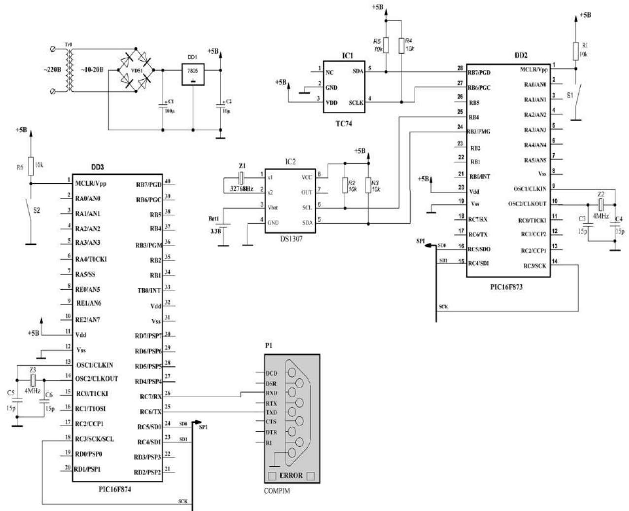
Рисунок 2.3 - Електрична принципова схема роботи Системи моніторингу температури
