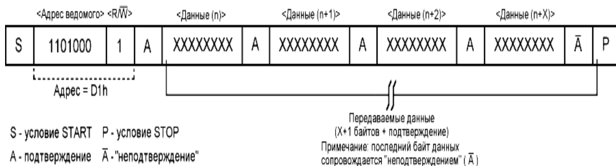
Рисунок 1.7 -Режим ведущего передатчика (режим чтения DS1307)
