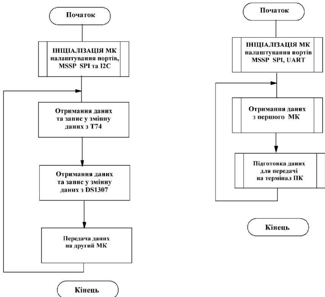
Рисунок 3.1 - Блок-схеми роботи Системи моніторингу температури
