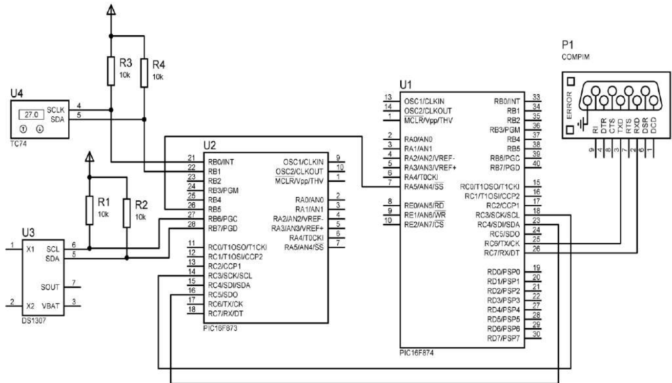
Рисунок 2.7 - Досліджувана схема
