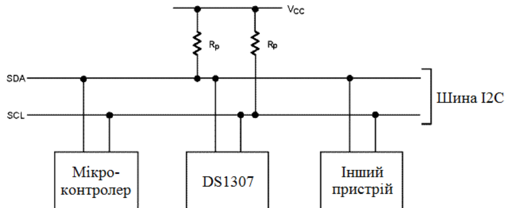
Рисунок 1.4 - Типова конфігурація двопровідної шини (I2C)
