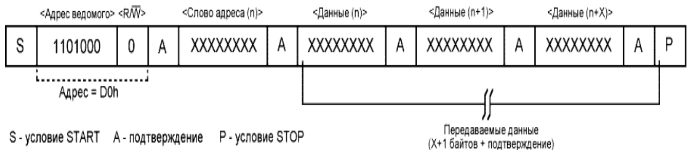
Рисунок 1.6 - Режим веденого приймача(режим запису DS1307).
