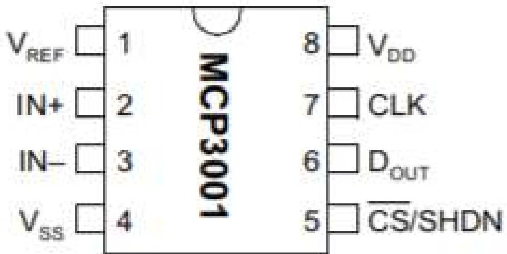
Рисунок 1.8 - Розпіновка приладу MCP3001
