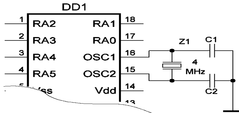
Рисунок 2.2 - Схема тактування мікроконтролера
