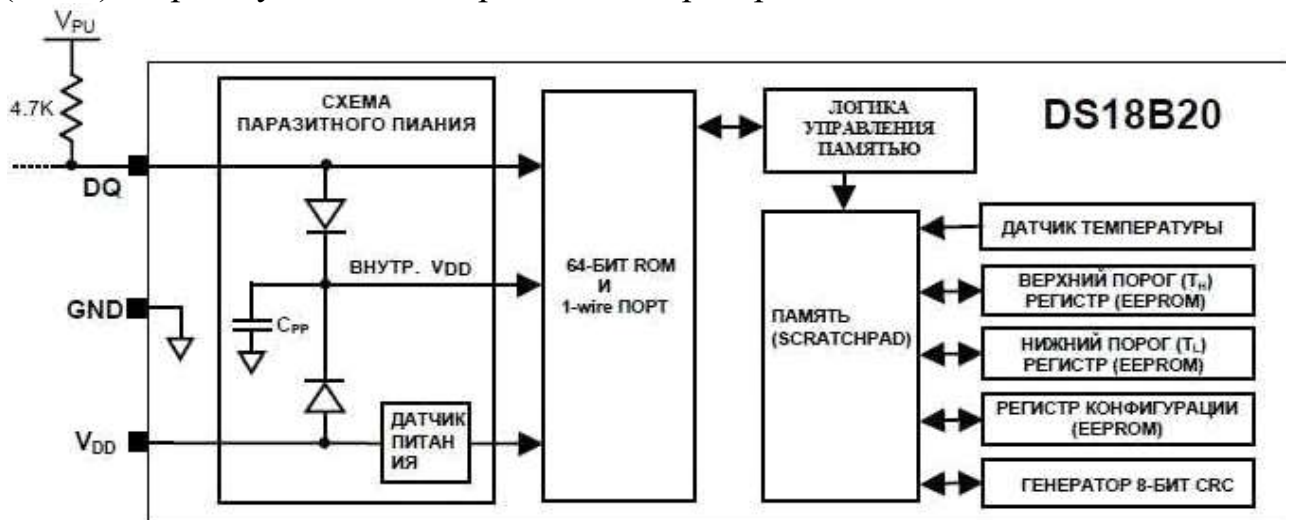
Рисунок 1.2- Блок-схема DS18B20
