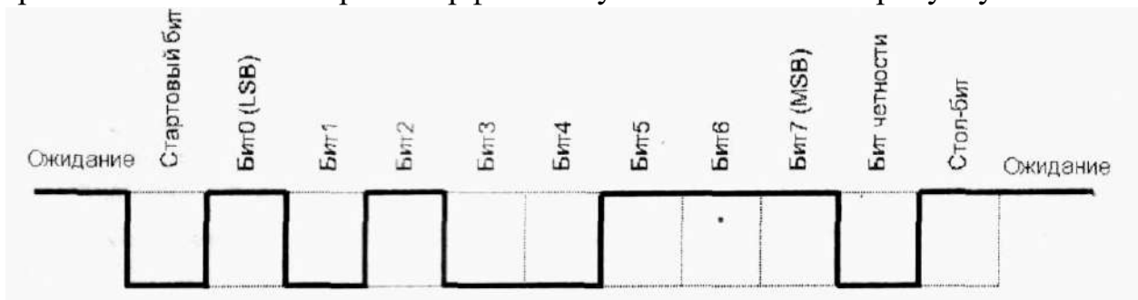
Рисунок 1.6 - Часова діаграма передачі байта E5h (11100101b).
