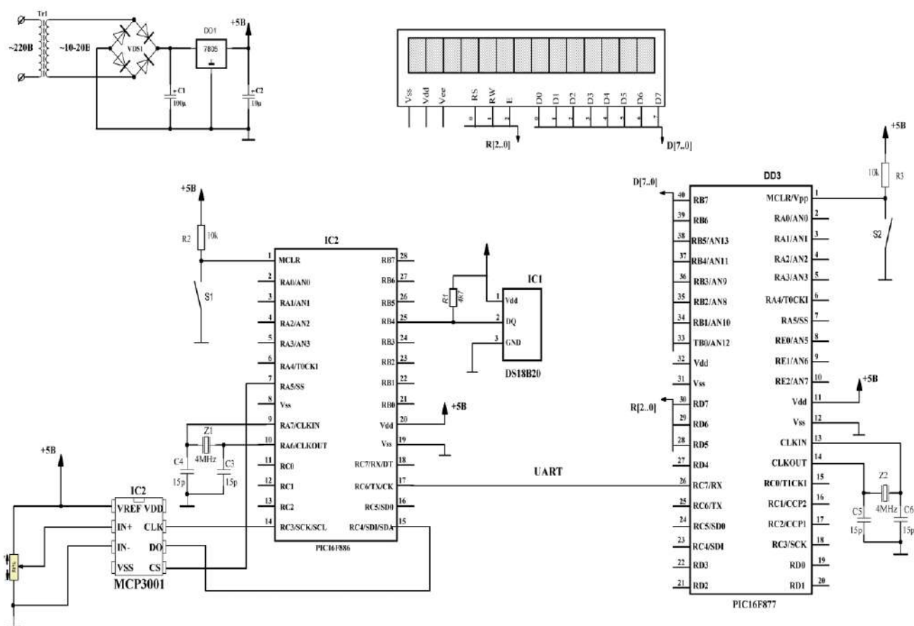
Рисунок 2.3 - Електрична принципова схема роботи Система моніторингу U та T
