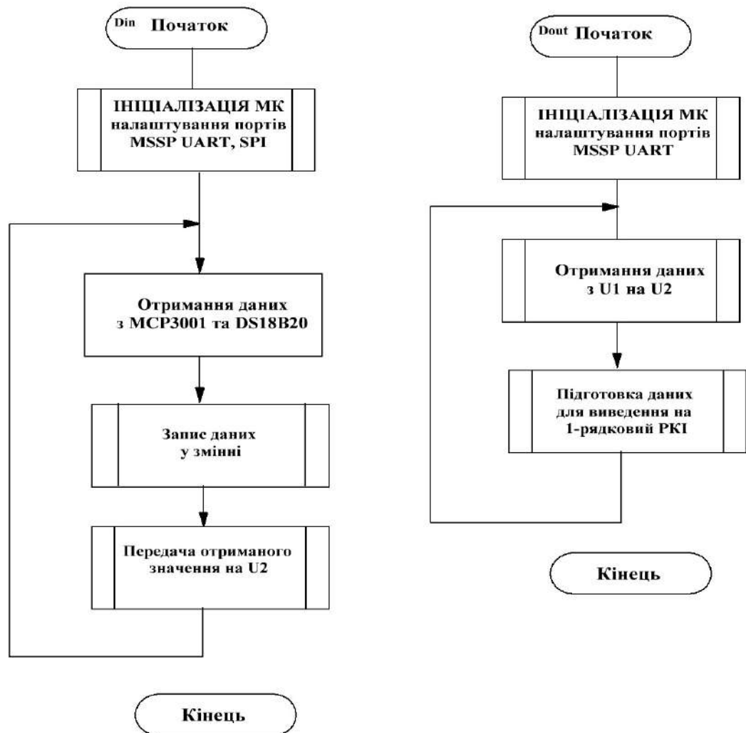
Рисунок 3.1 - Блок-схеми роботи Система моніторингу U та T
