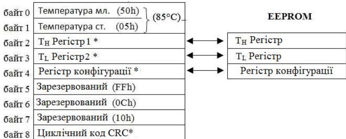
Рисунок 1.3 - Карта пам'яті DS18B20
