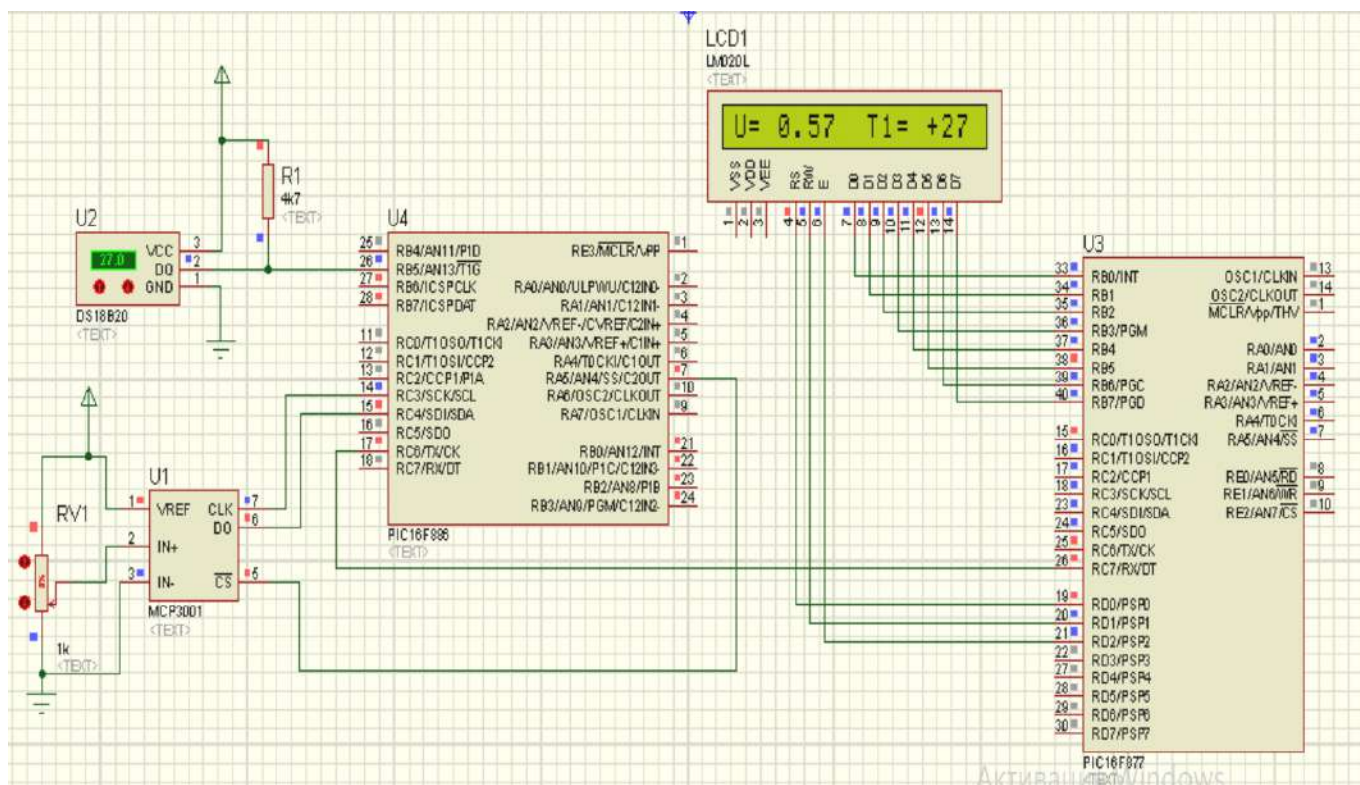
Рисунок 3.2 - Робоча схеми в PROTEUS
