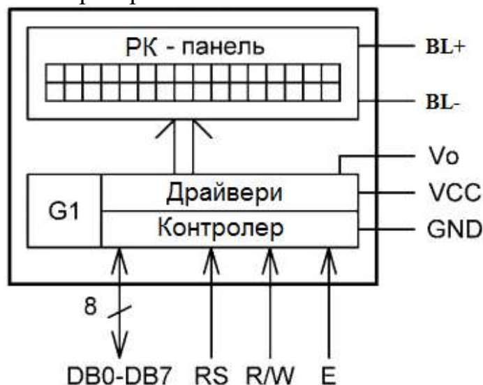
Рисунок 1.4 – Структурна схема РКІ
