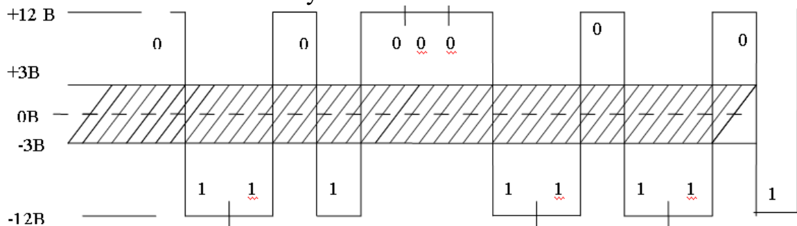
Рисунок 1.5 - Реалізація інтерфейсу RS-232 на фізичному рівні
