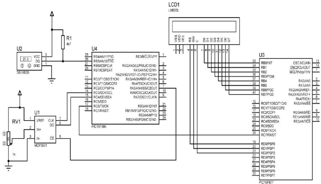
Рисунок 2.7 - Досліджувана схема
