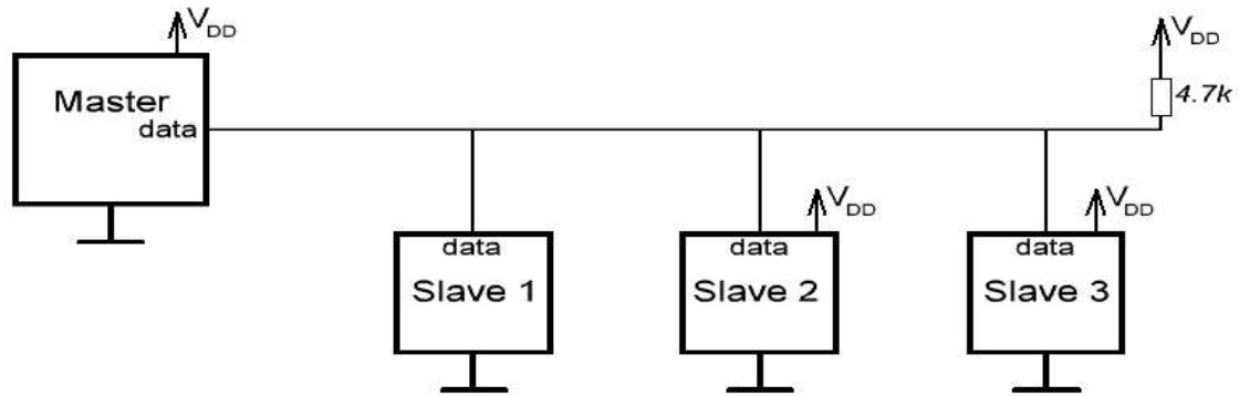
Рисунок 1.7 -Приклад підключення ведучого і ведених приладів за протоколом 1-Wire
