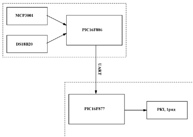
Рисунок 1.1 - Структурна схема Система моніторингу U та T
