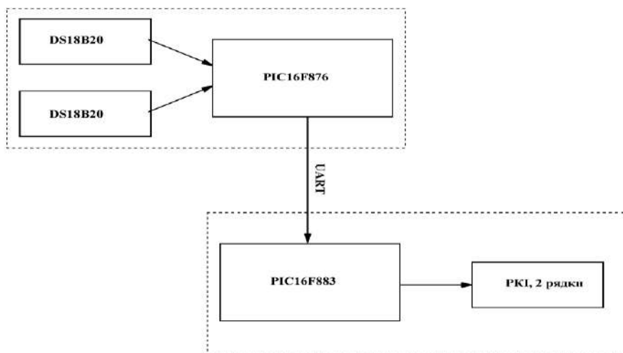
Рисунок 1.1 - Структурна схема системи моніторингу температури
