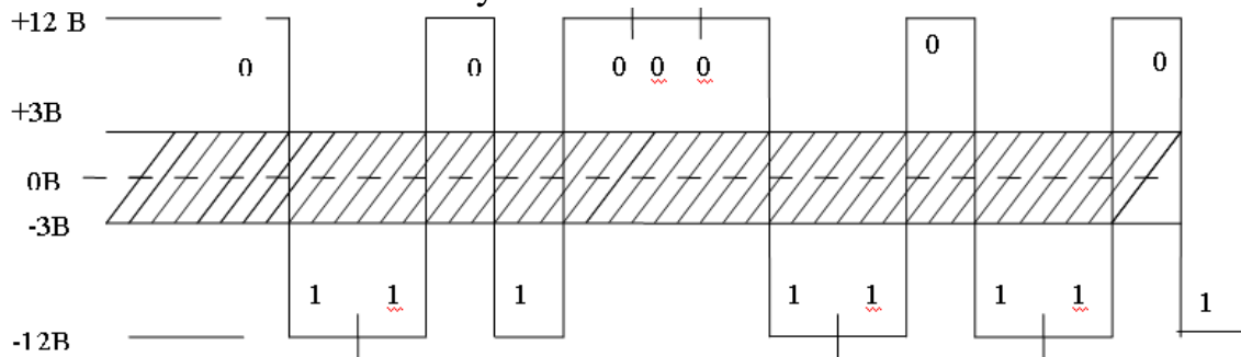
Рисунок 1.7 - Реалізація інтерфейсу RS-232 на фізичному рівні
