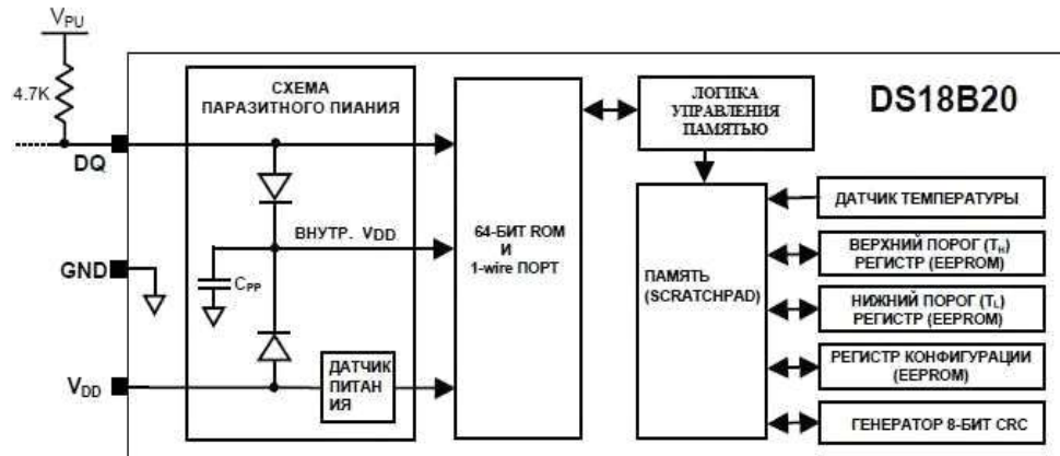
Рисунок 1.2- Блок-схема DS18B20
