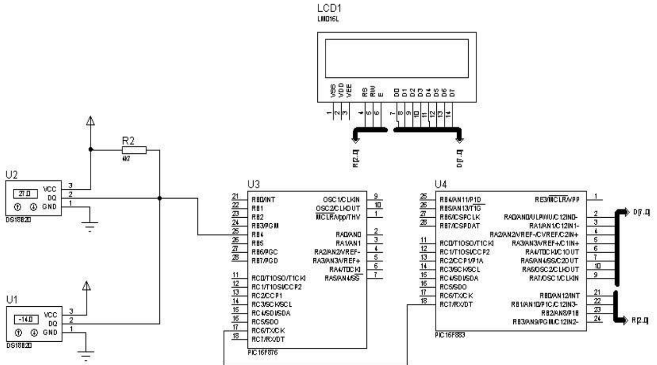
Рисунок 2.7 – Досліджувана схема
