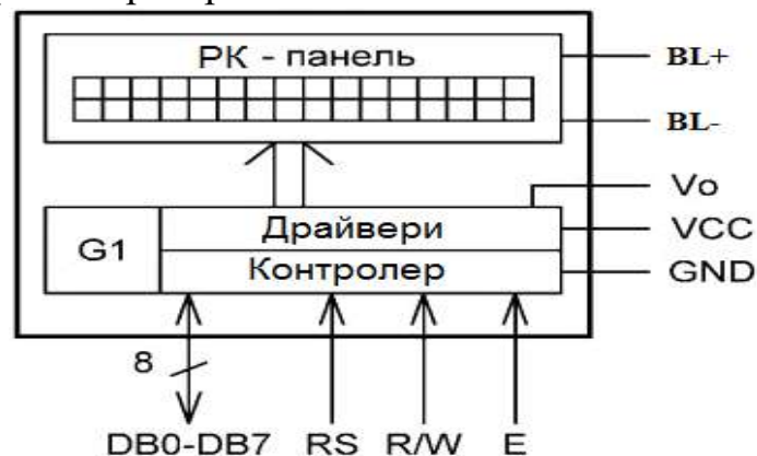
Рисунок 1.4 – Структурна схема РКІ
