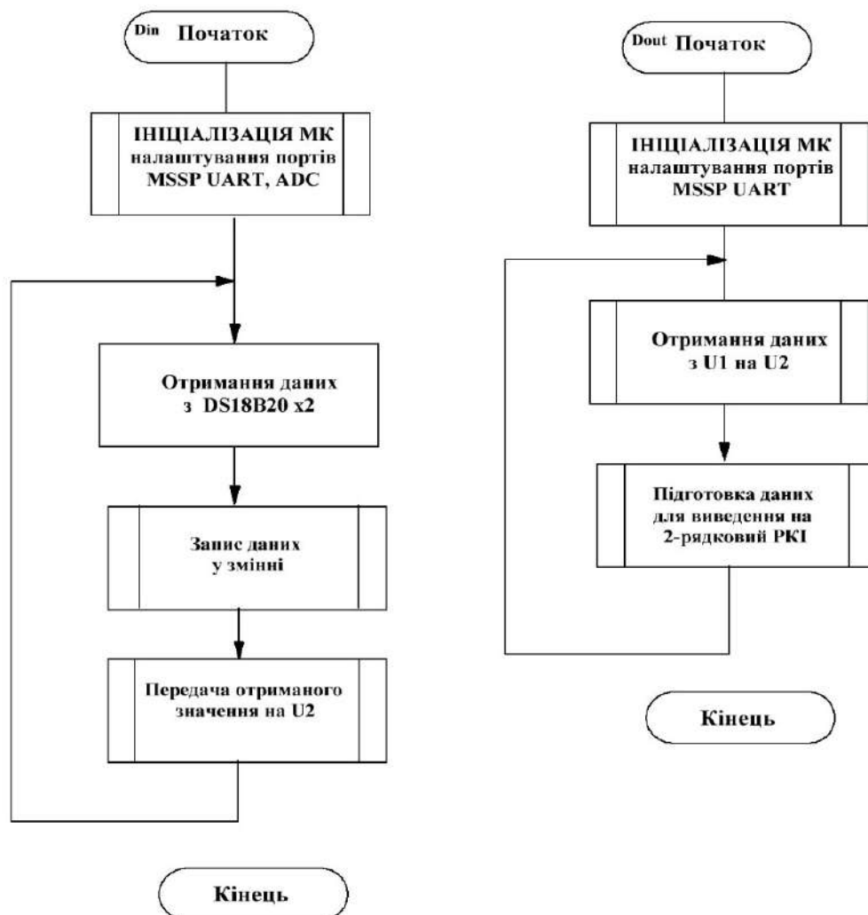
Рисунок 3.1 - Блок-схеми роботи Система моніторингу температури
