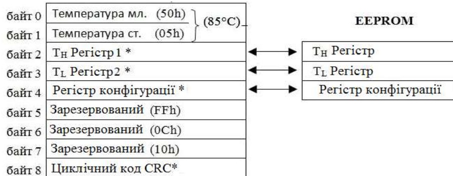
Рисунок 1.3 - Карта пам'яті DS18B20
