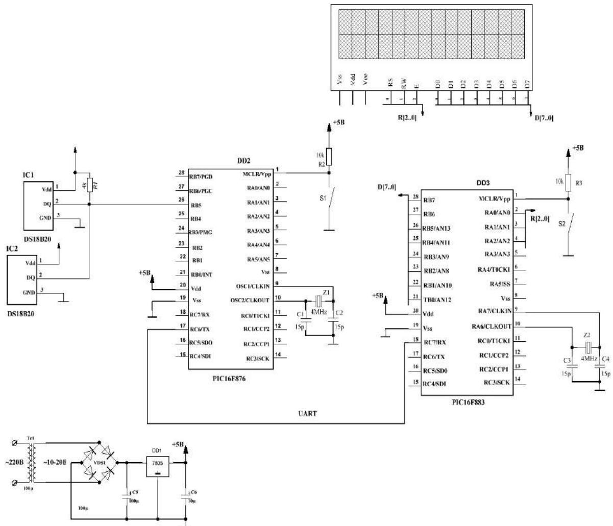
Рисунок 2.3 - Електрична принципова схема роботи Системи моніторингу температури
